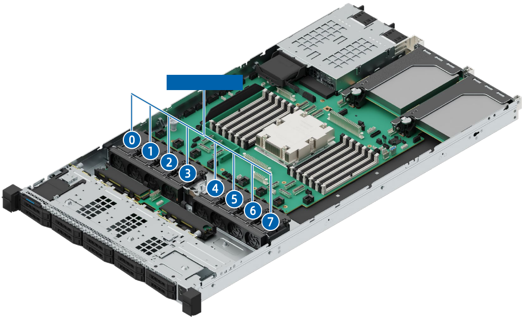
图 5-18 风扇模块的位置
