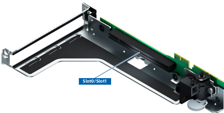
图 5-14 PCIe 转接卡模组 0/1 (1 个 x16 插槽)
