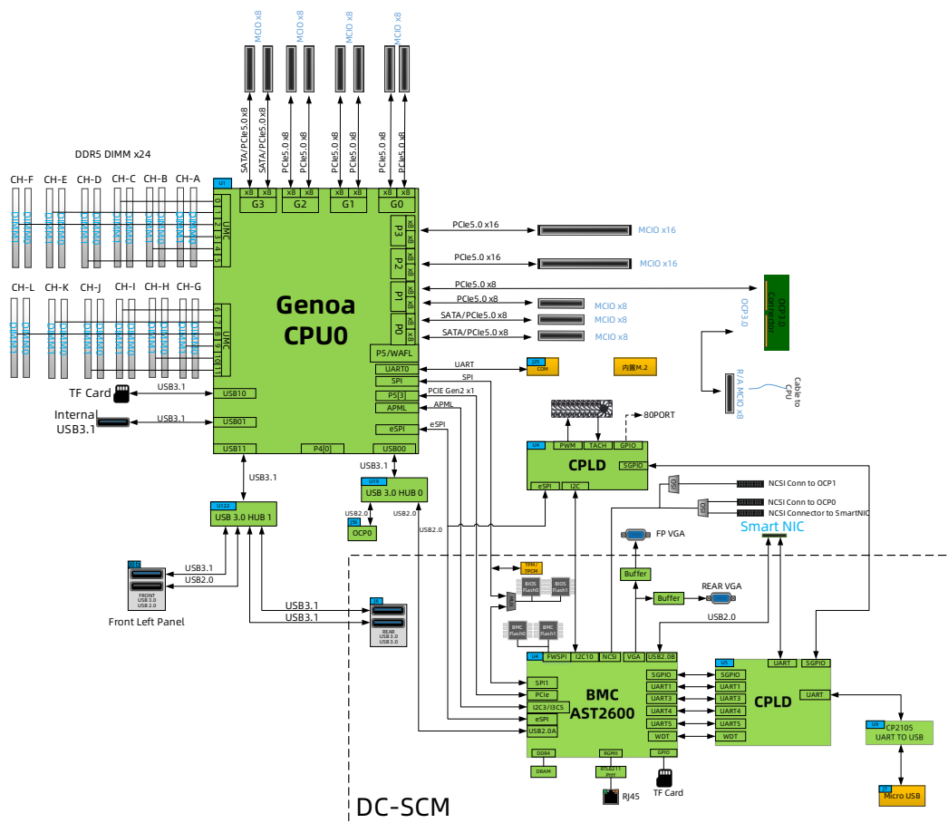
图 4-1 NF3180G7 逻辑结构
