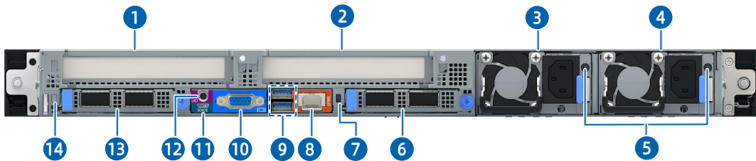
图 5-3 2 × PCIe 插槽后面板外观
