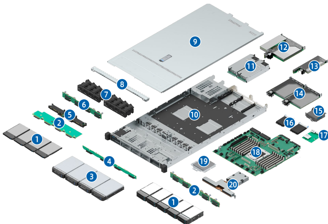
图 3-1 NF3180G7 物理结构
