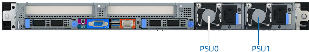
图 5-17 电源模块位置
