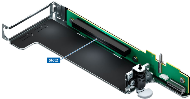
图 5-16 PCIe 转接卡模组 3 (1 个 x16 插槽)
