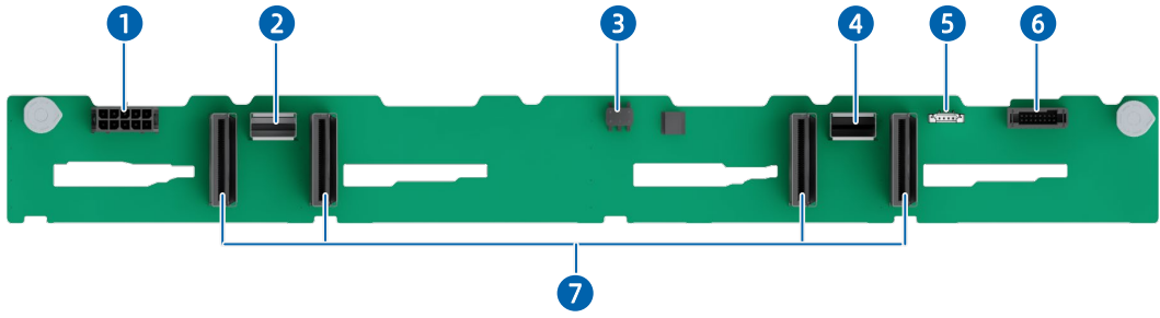
图 5-23 8 × 2.5 英寸 (SAS/SATA/NVMe) 硬盘背板
