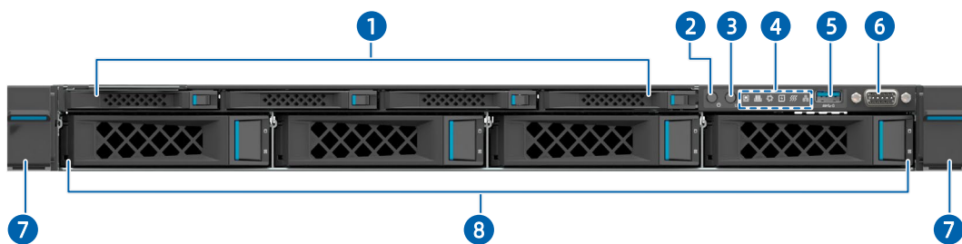
图 5-1 4 × 2.5 英寸硬盘+4 × 3.5 英寸硬盘前面板外观
