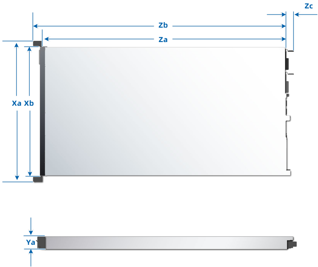
图 6-1 主机尺寸
