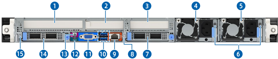
图 5-4 3 × PCIe 插槽后面板外观
