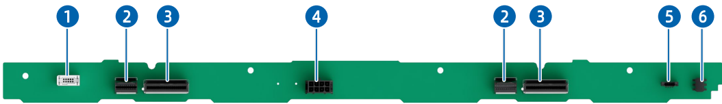
图 5-21 4 × 3.5 英寸 (SAS/SATA/NVMe) 硬盘背板
