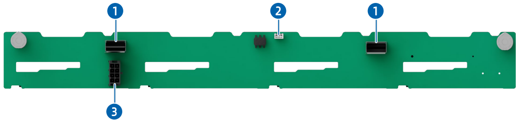
图 5-24 8 × 2.5 英寸 (SAS/SATA) 硬盘背板
