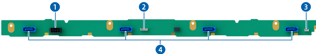
图 5-22 4 × 3.5 英寸 (SAS/SATA) 硬盘背板
