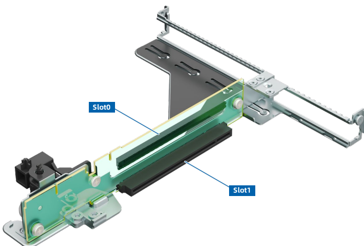
图 5-15 PCIe 转接卡模组 2 (2 个 x16 插槽)
