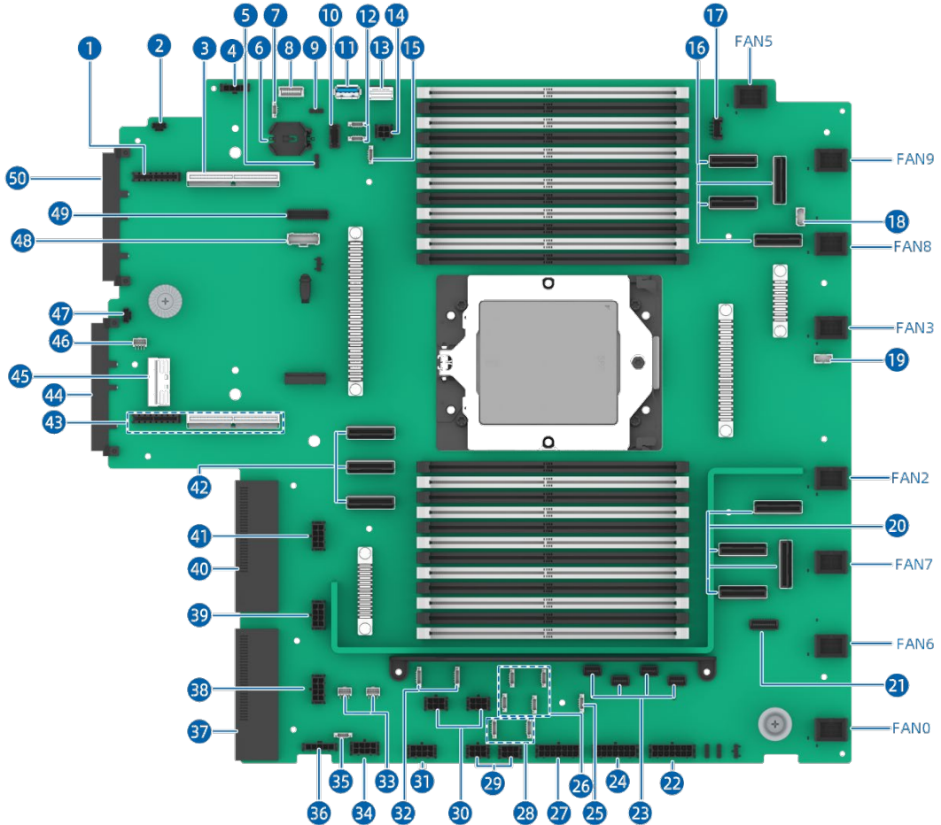
图 5-19 主板
