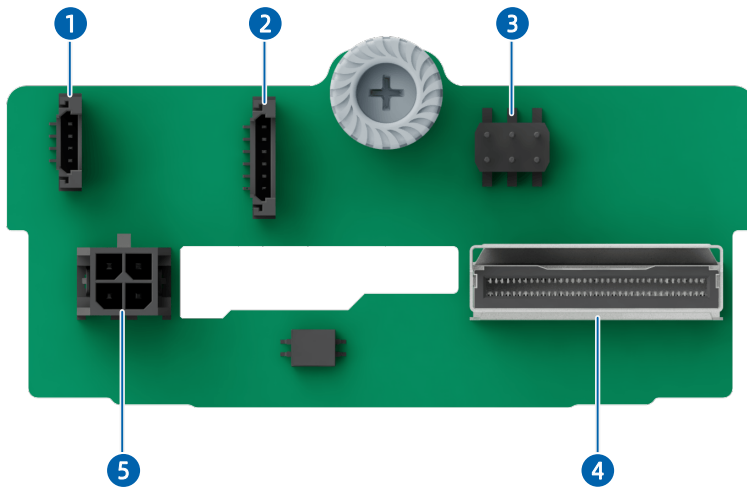
图 5-26 2 × 2.5 英寸 (NVMe) 硬盘背板
