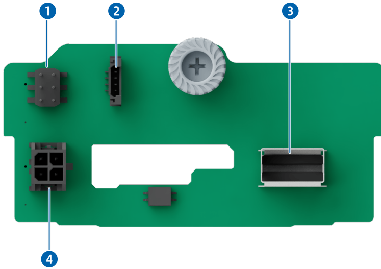
图 5-25 2 × 2.5 英寸 (SAS/SATA) 硬盘背板
