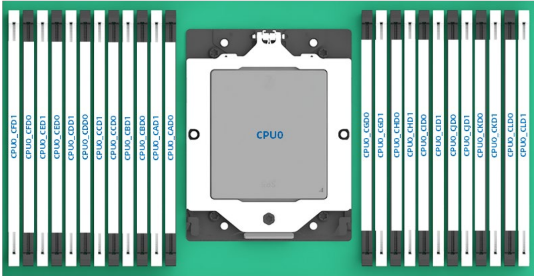
图 5-7 内存插槽位置
