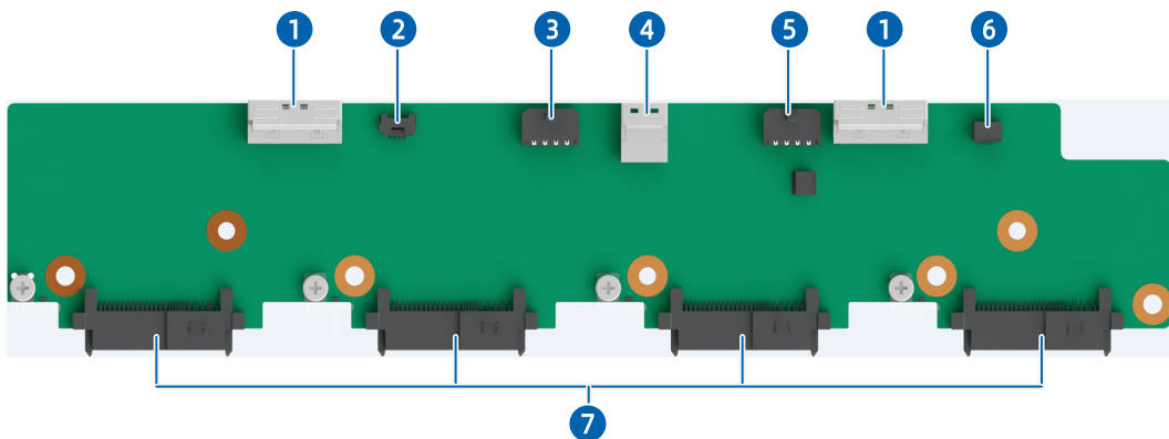
图 5-20 4 × 2.5 英寸 (SAS/SATA/NVMe) 硬盘背板
