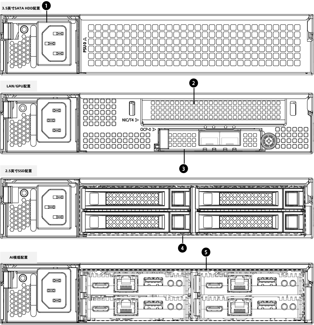
图 5-7 后面板示意图
