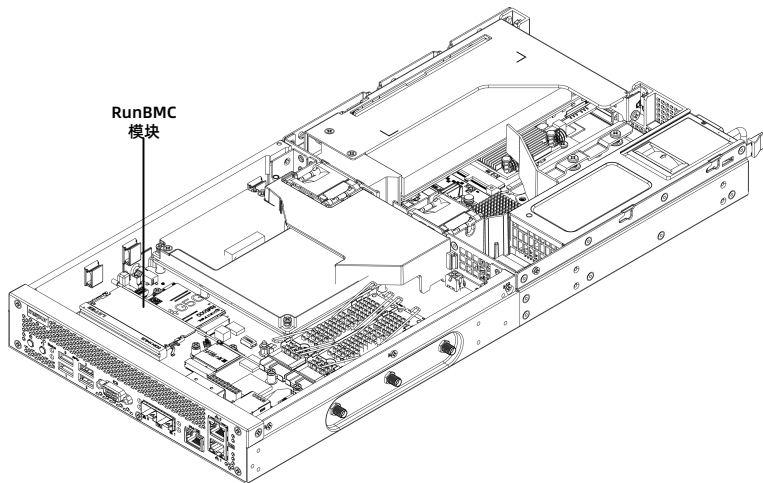
图 5-21 RunBMC 位置示意图
