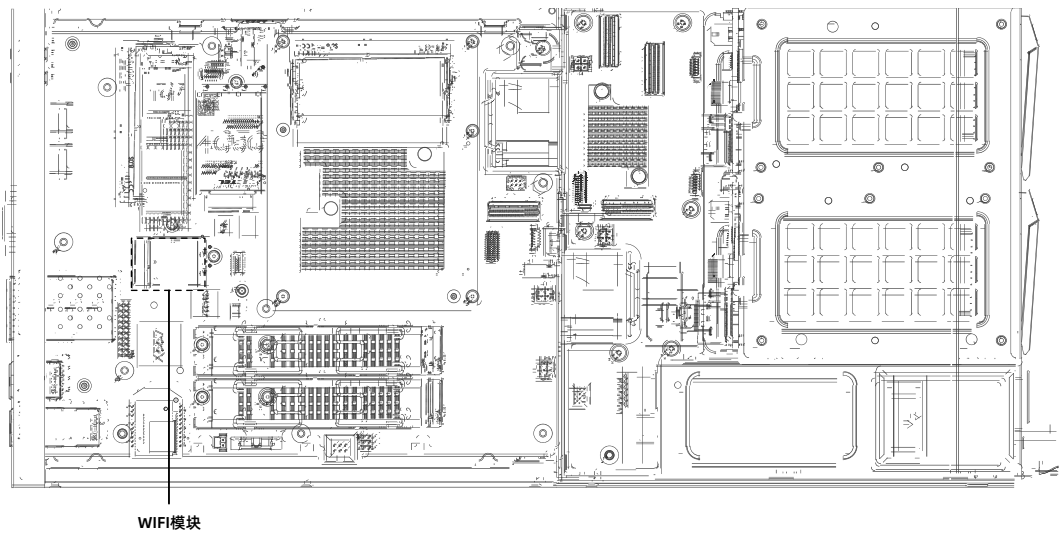
图 5-19 模块安装位置
