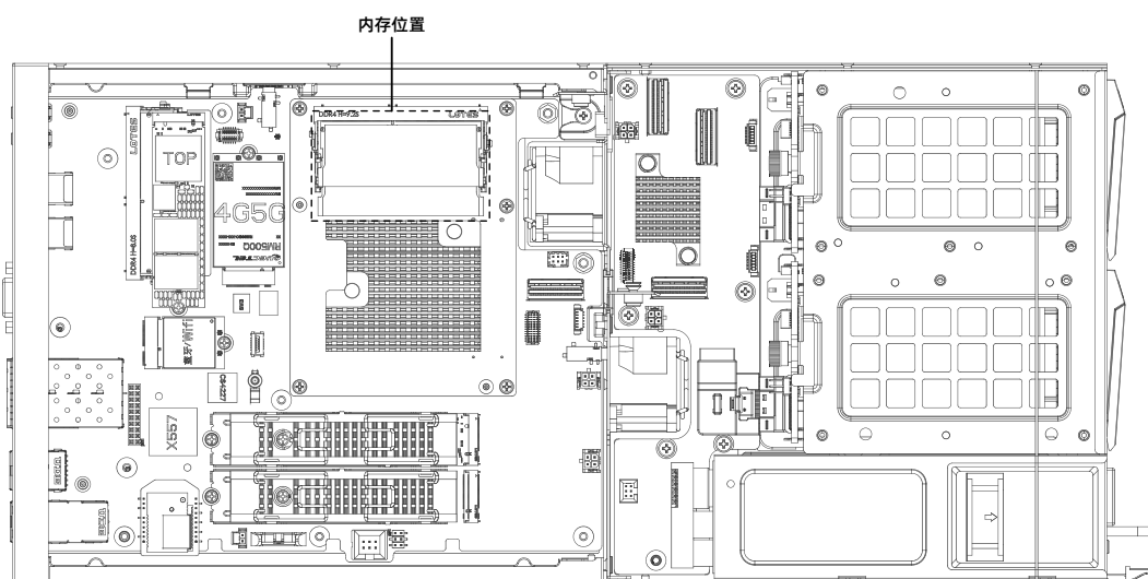
图 5-15 内存插槽位置
