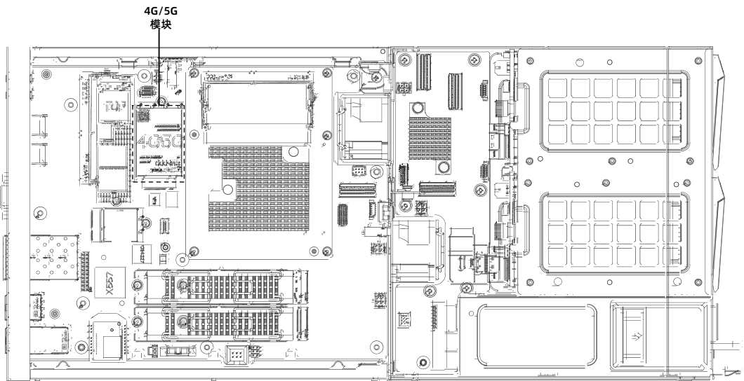
图 5-18 模块安装位置
