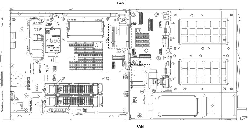
图 5-26 EIS800E 风扇模块的位置
