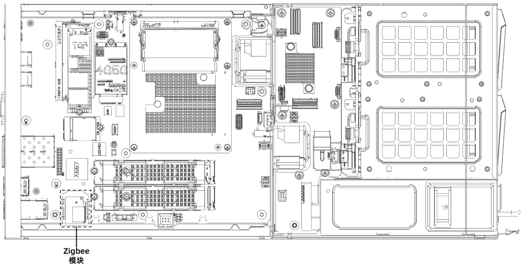
图 5-20 Zigbee 模块安装位置
