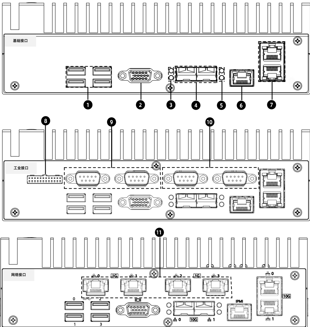
图 5-2 前面板示意图
