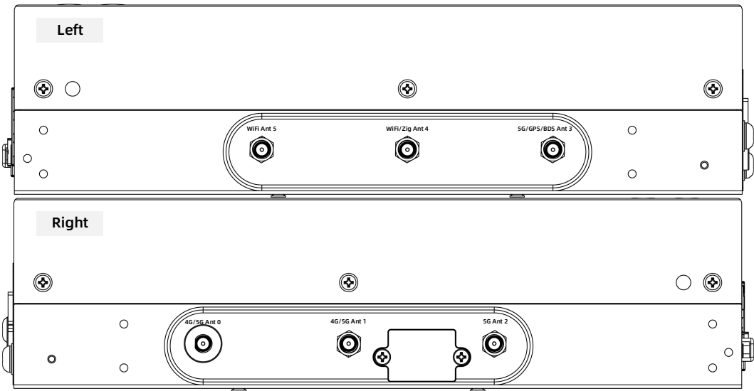
图 5-8 侧面板示意图
