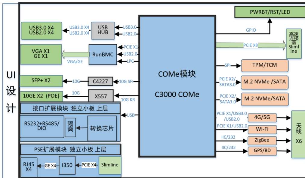
图 4-1 EIS800S 的逻辑结构
