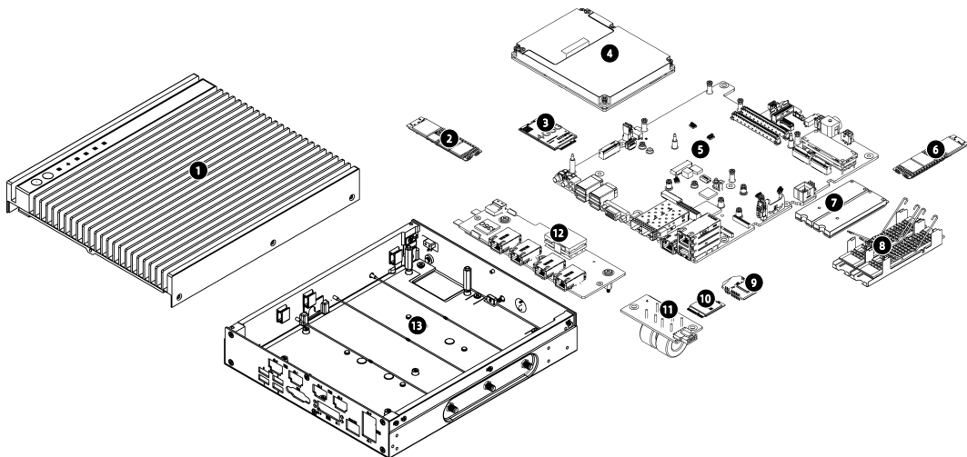
图 5-1 EIS800S 爆炸图
