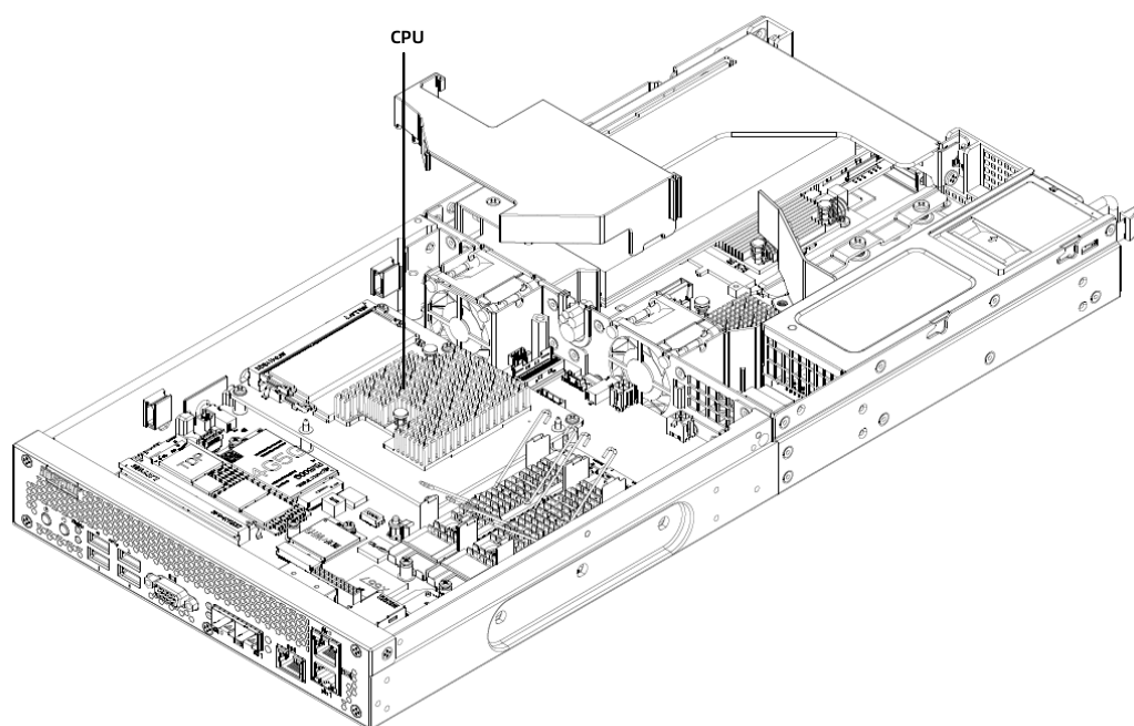
图 5-13 处理器位置示意图
