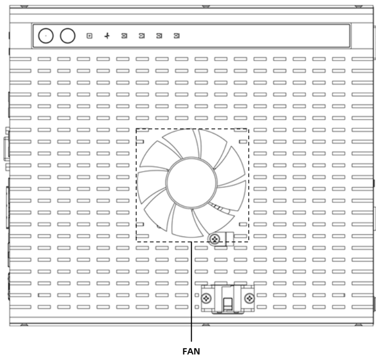
图 5-25 EIS800S 带风扇机型风扇模块的位置
