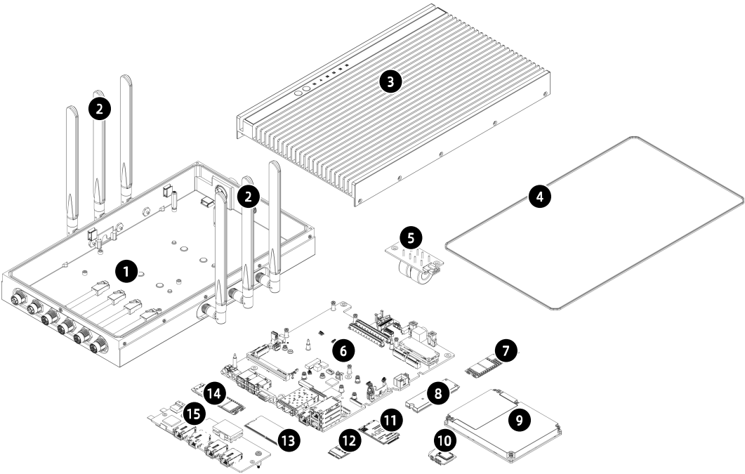
图 5-9 EIS800P 爆炸图
