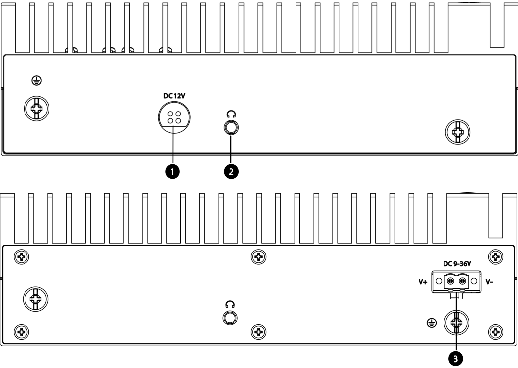
图 5-3 后面板示意图
