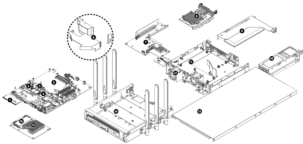
图 5-5 EIS800E 爆炸图
