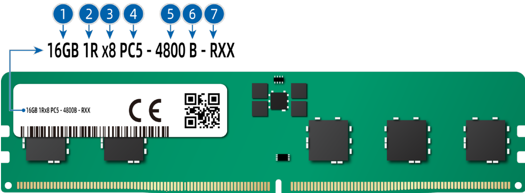
图 5-5 内存标识
