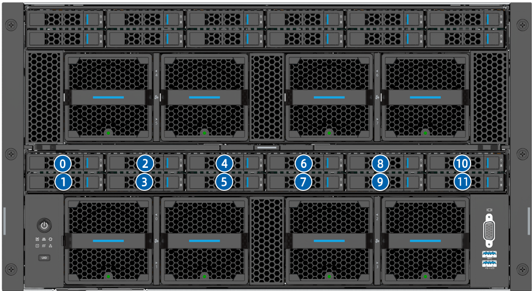
图 5-8 TS860-M7-A0-R0-00 硬盘编号（搭配 16i RAID 控制卡）
