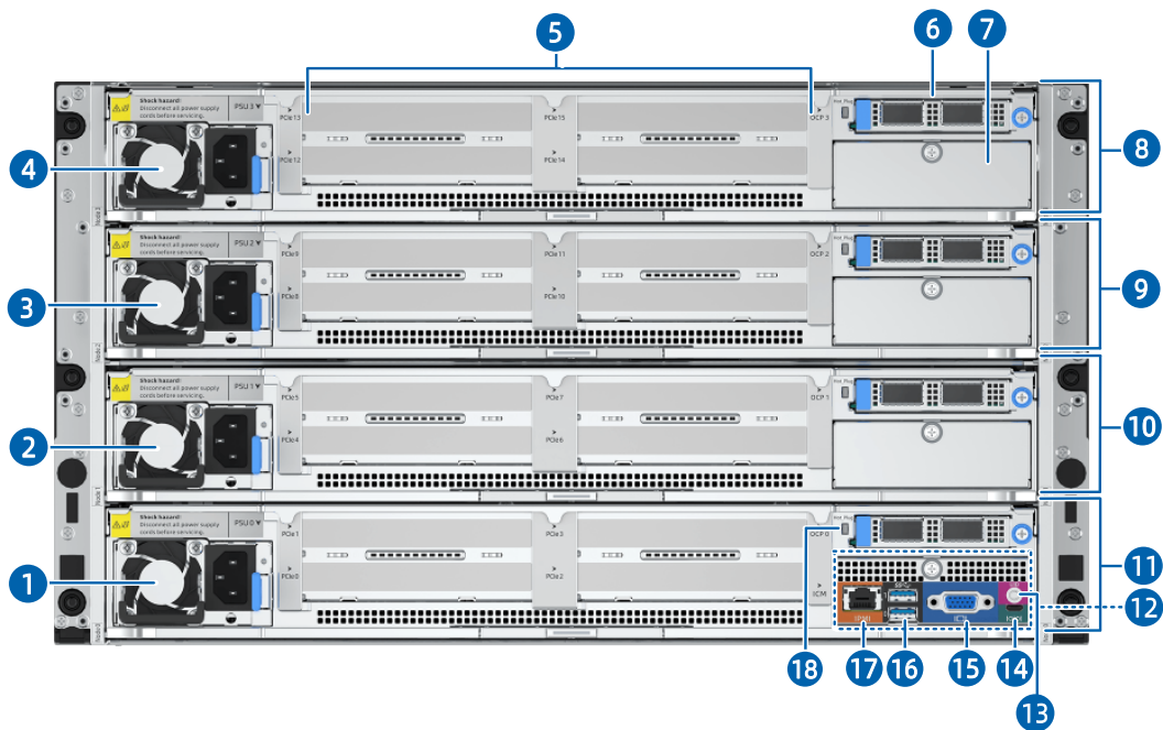
图 5-2 16 × PCIe 插槽后视图
