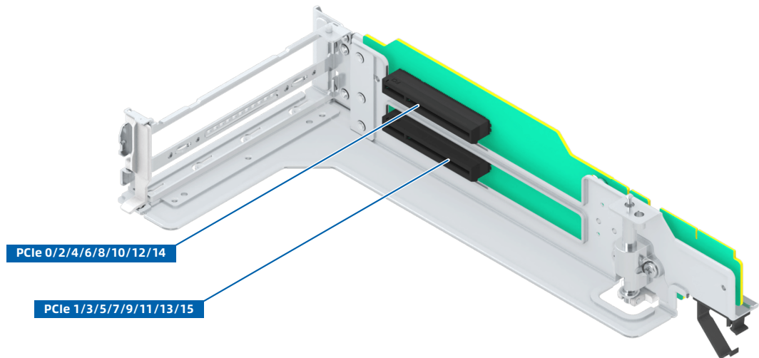
图 5-15 槽位标识（2 个 x8 插槽）
