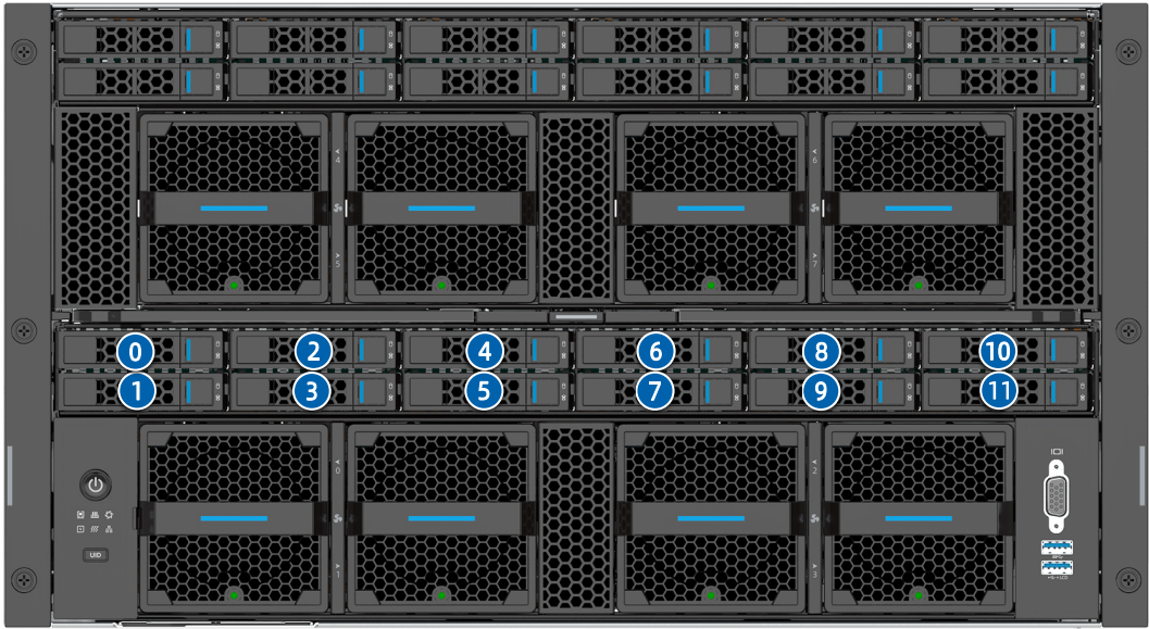
图 5-7 TS860-M7-A0-R0-00 硬盘编号（搭配 8i RAID 控制卡）
