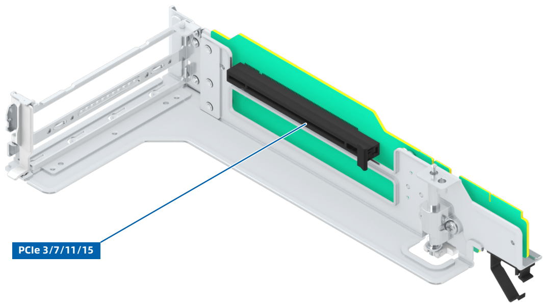
图 5-17 槽位标识（1 个 x16 插槽）
