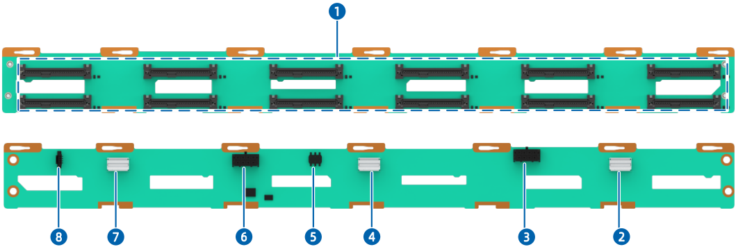
图 5-26 12 × 2.5 英寸硬盘配置（12 × SAS/SATA）背板
