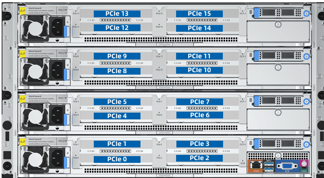
图 5-13 16 × PCIe 配置
