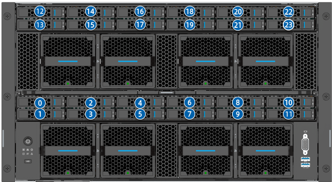
图 5-9 TS860-M7-A0-R0-00 硬盘编号
