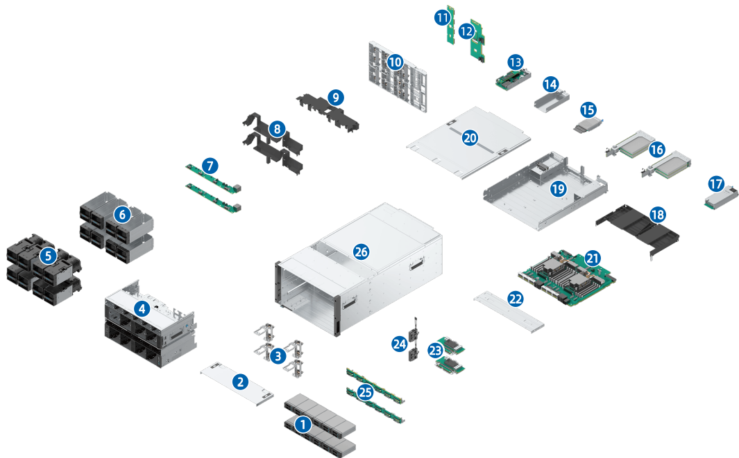
图 3-1 TS860G7 系列服务器物理结构（以 24 × 2.5 英寸硬盘配置为例）
