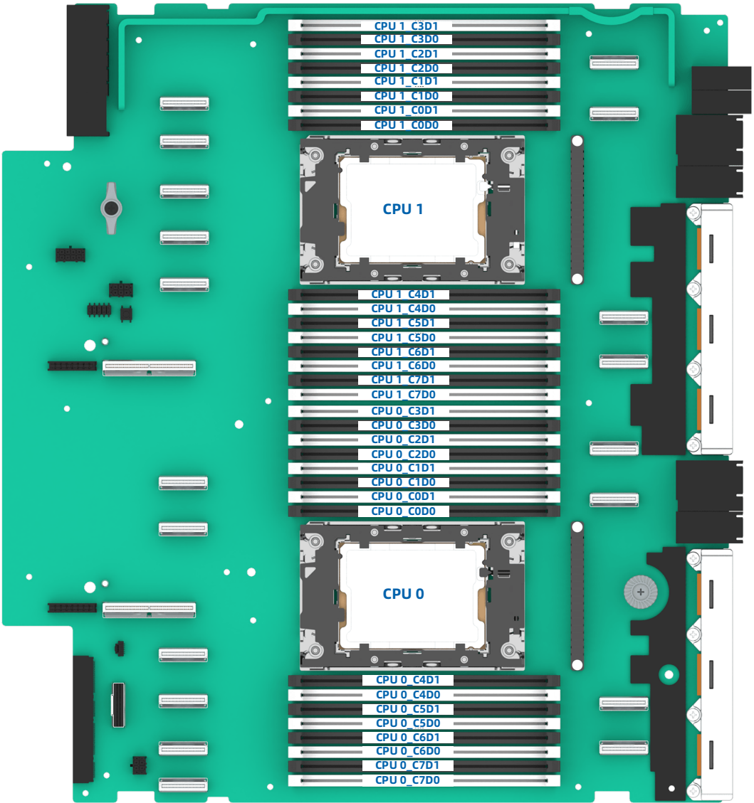
图 5-6 内存插槽布局（以节点 0 为例）
