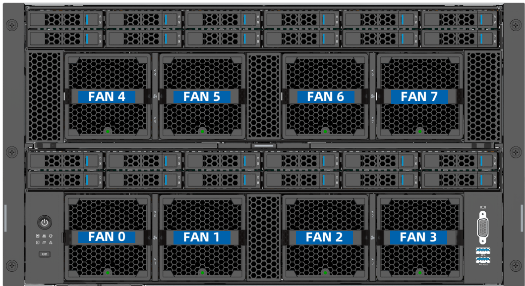
图 5-20 风扇模组的位置
