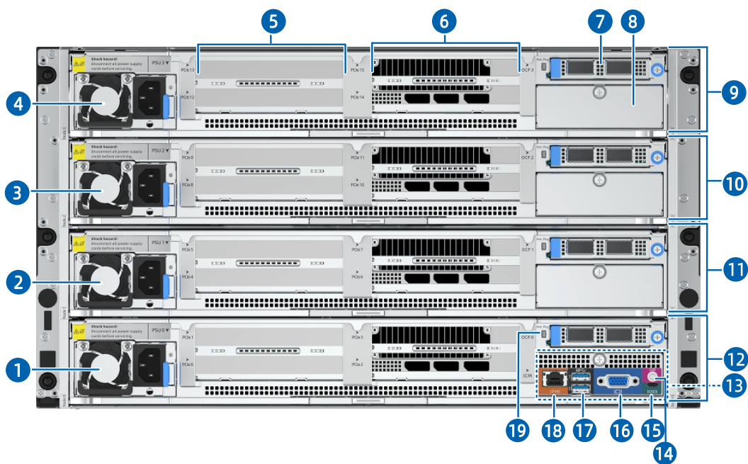
图 5-3 8 × PCIe+4 × GPU 插槽后视图
