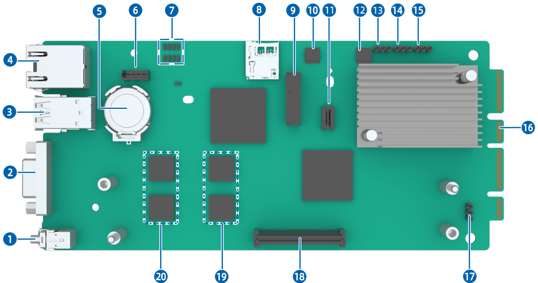
图 5-25 ICM 板
