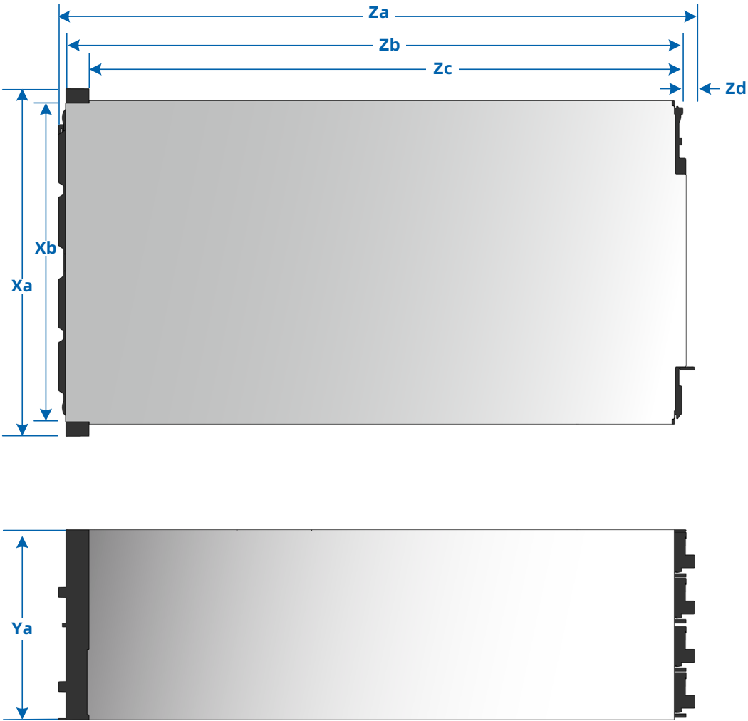
图 6-1 主机尺寸
