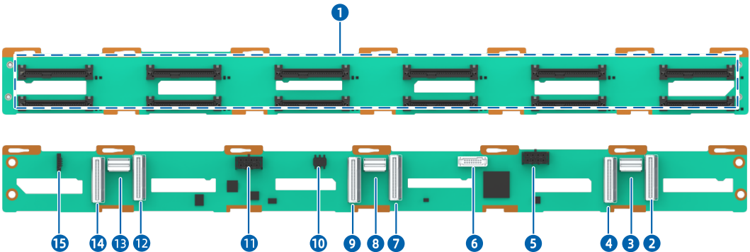
图 5-27 12 × 2.5 英寸硬盘配置（12 × SAS/SATA/NVMe）背板
