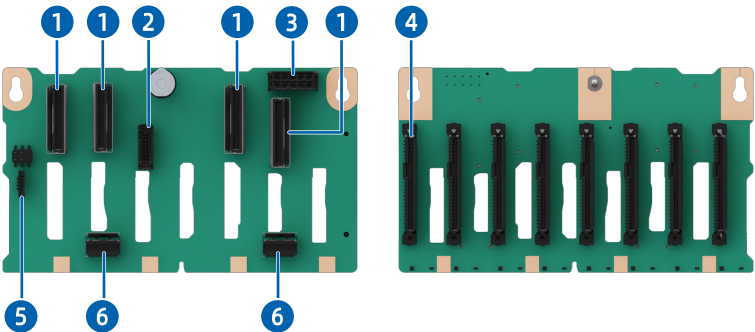
图 5-59 8 × 2.5 英寸硬盘配置 (8 × SAS/SATA/NVMe) 背板
