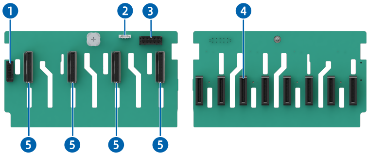
图 5-61 8 × 2.5 英寸硬盘配置 (8 × NVMe) 背板
