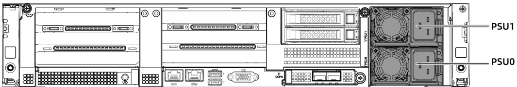
图 5-16 电源模块位置
