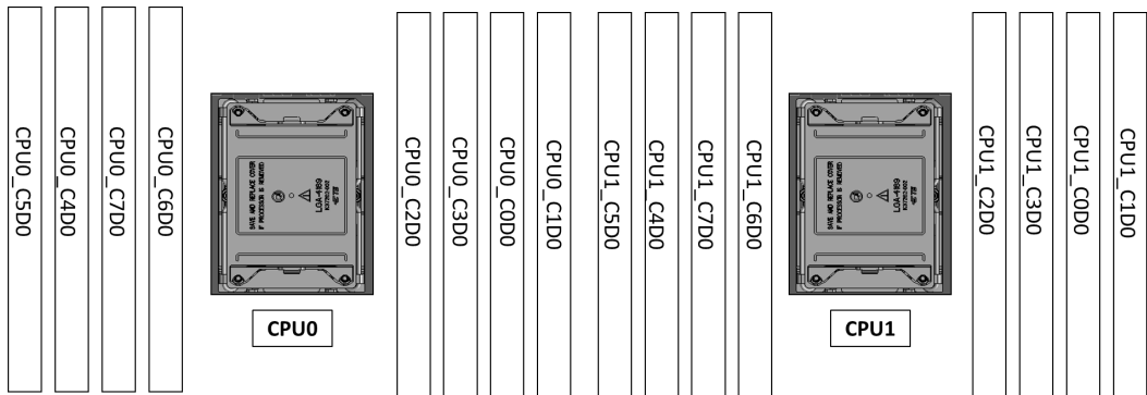
图 5-9 内存插槽位置
