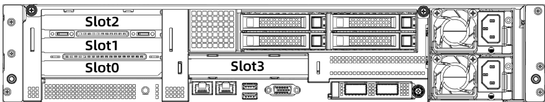
图 5-14 PCIe 插槽-4PCIe 配置
