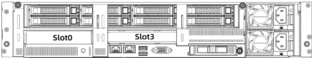
图 5-15 PCIe 插槽-2PCIe 配置
