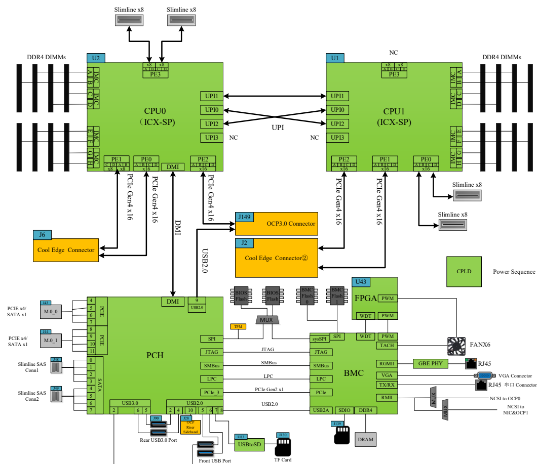
图 4-1 NF5266M6 逻辑结构
