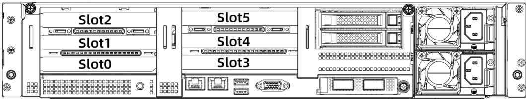
图 5-12 PCIe 插槽-6PCIe 配置
