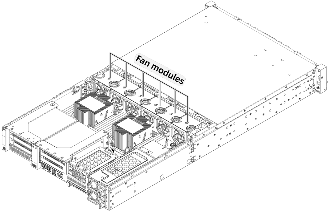
图 5-17 风扇模块的位置
