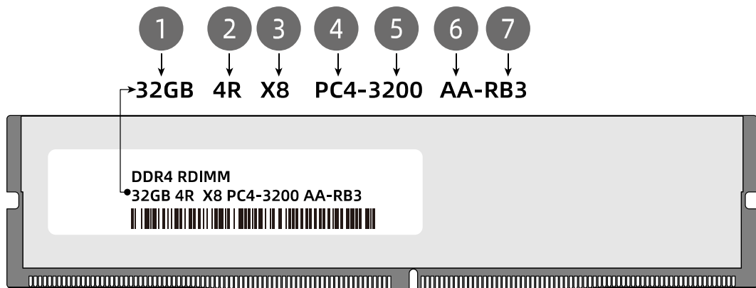
图 5-6 内存标识
