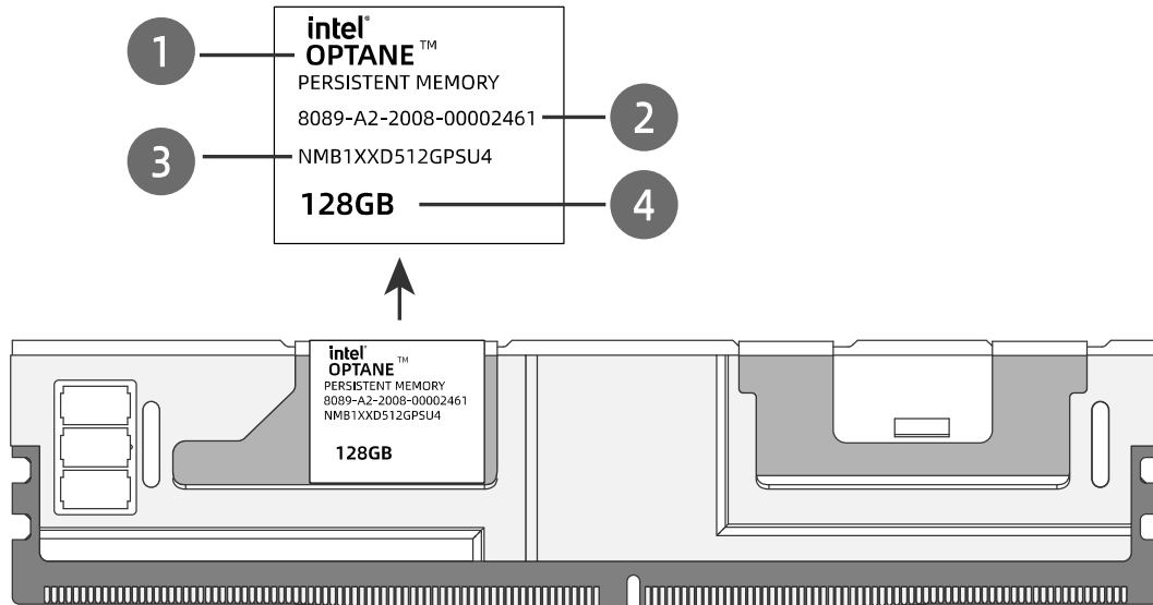
图 5-8 内存标识
