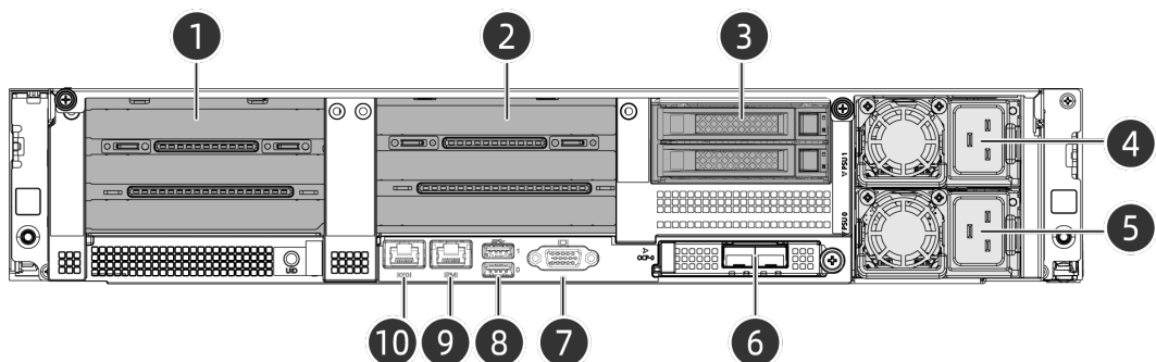
图 5-3 后面板外观
