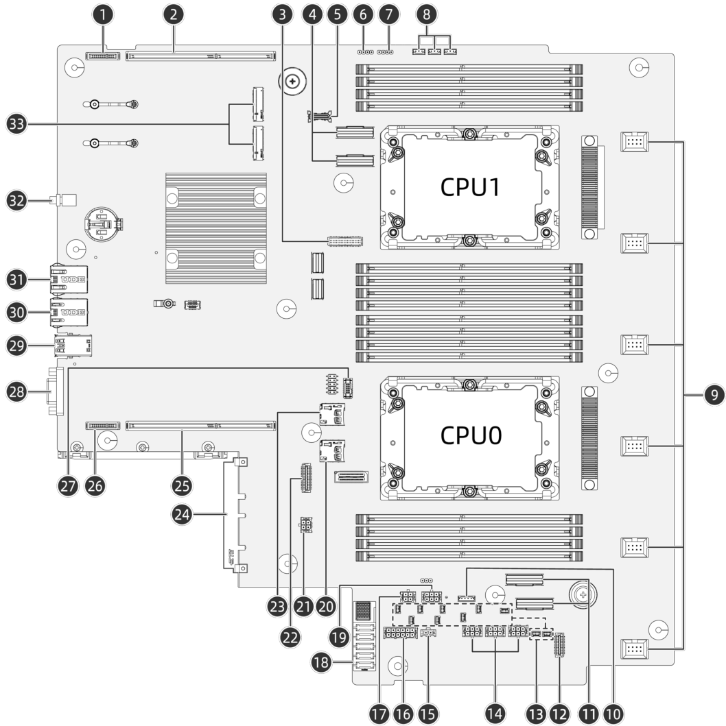
图 5-18 主板
