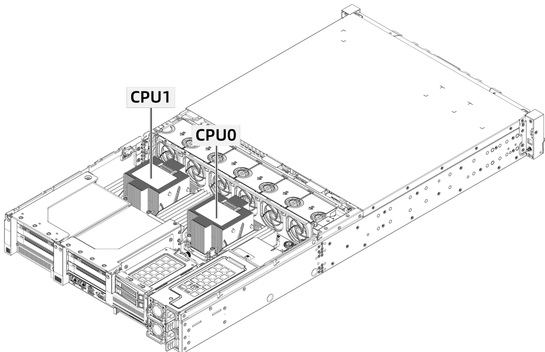
图 5-5 处理器位置
