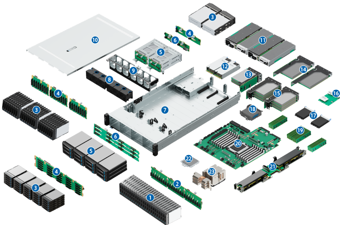
图 3-1 NF3280G7 物理结构
