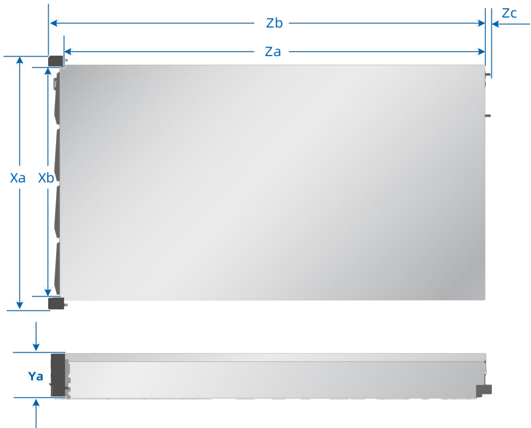
图 6-1 主机尺寸
