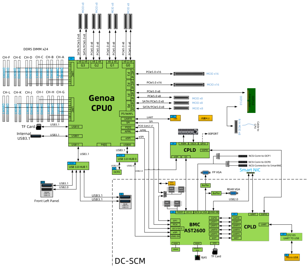
图 4-1 NF3280G7 逻辑结构
