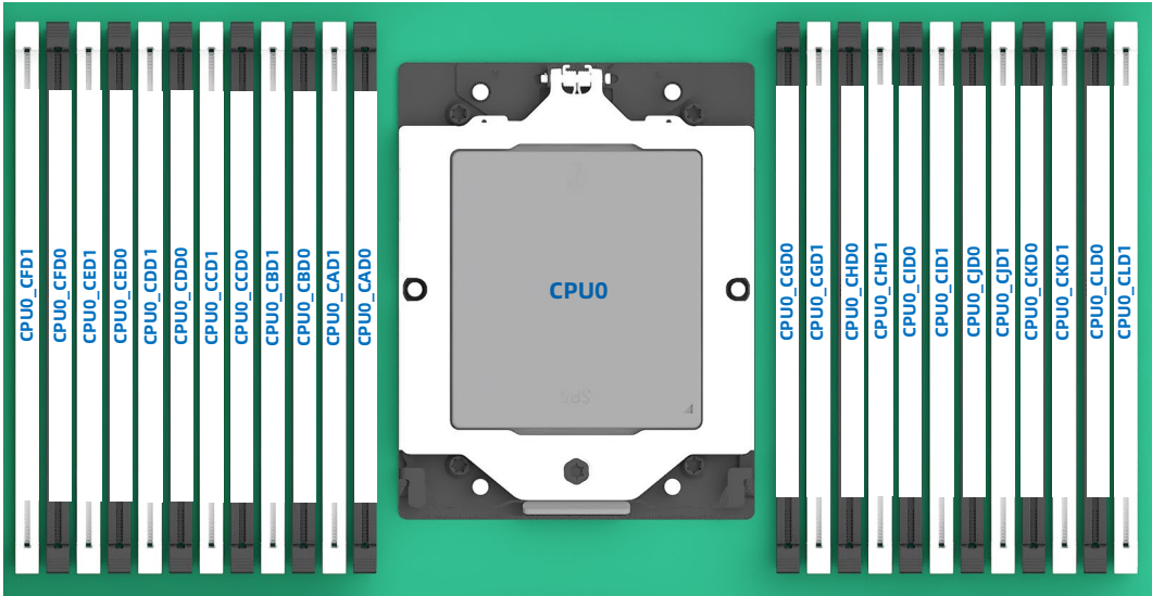
图 5-12 内存插槽位置
