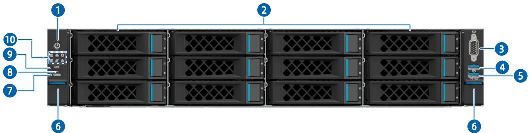
图 5-3 12 × 3.5 英寸硬盘配置前面板外观
