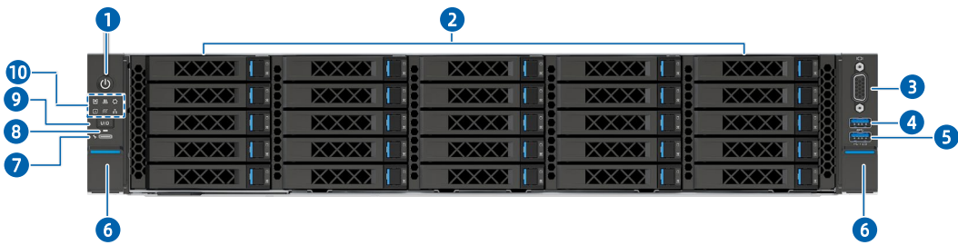
图 5-2 25 × 2.5 英寸硬盘配置前面板外观
