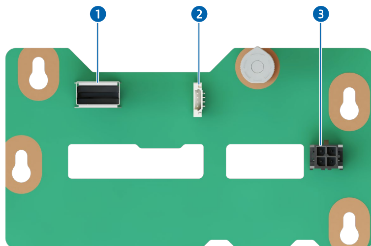
图 5-34 2 × 3.5 英寸 (SAS/SATA) 硬盘背板
