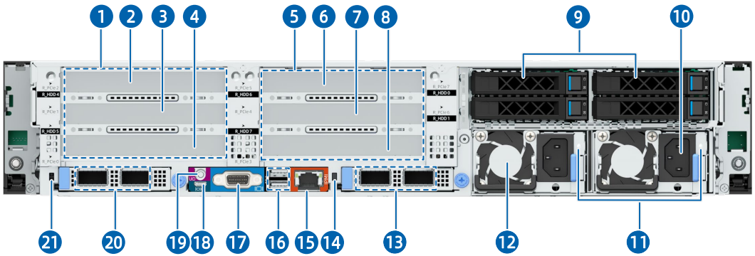
图 5-8 4 × 2.5 英寸硬盘+6 × PCIe 插槽配置后面板外观
