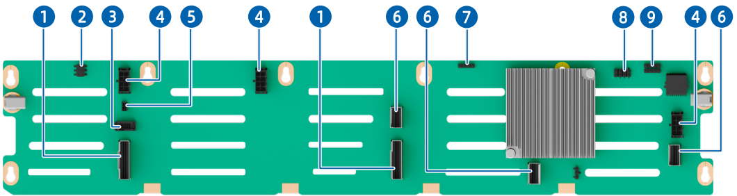
图 5-29 25 × 2.5 英寸（SAS/SATA/NVMe）硬盘背板
