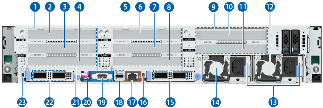
图 5-5 8 × PCIe 插槽配置后面板外观
