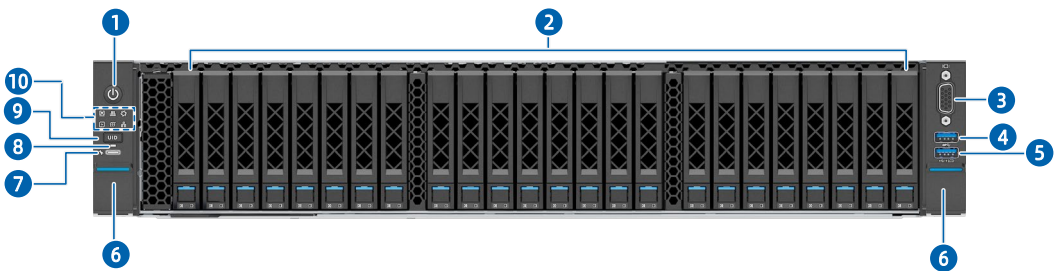
图 5-1 24 × 2.5 英寸硬盘配置前面板外观
