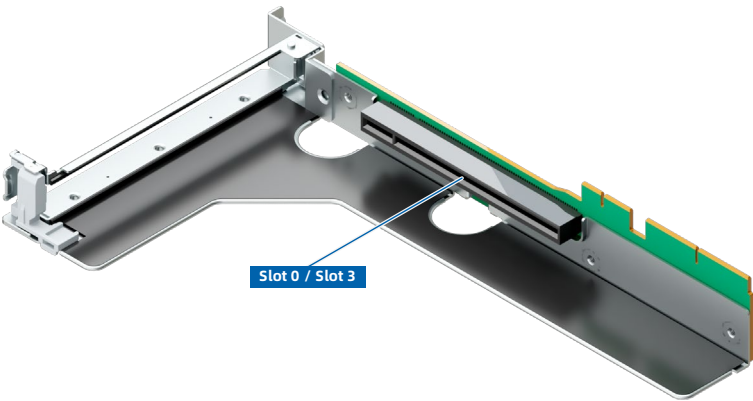
图 5-24 PCIe 转接卡模组 3/4 (1 个 x16 插槽)
