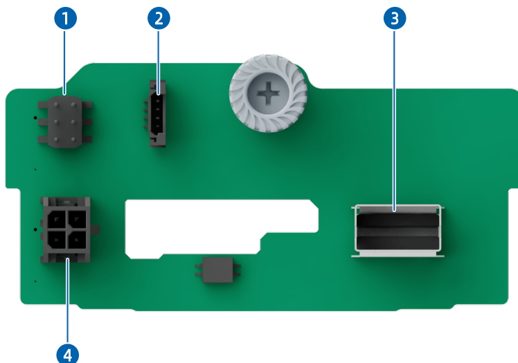
图 5-35 2 × 2.5 英寸 (SAS/SATA) 硬盘背板
