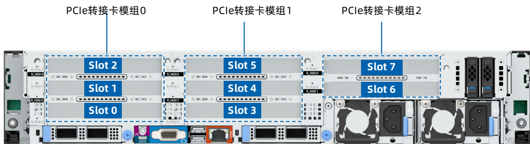
图 5-20 PCIe 插槽-8 × PCIe 插槽配置
