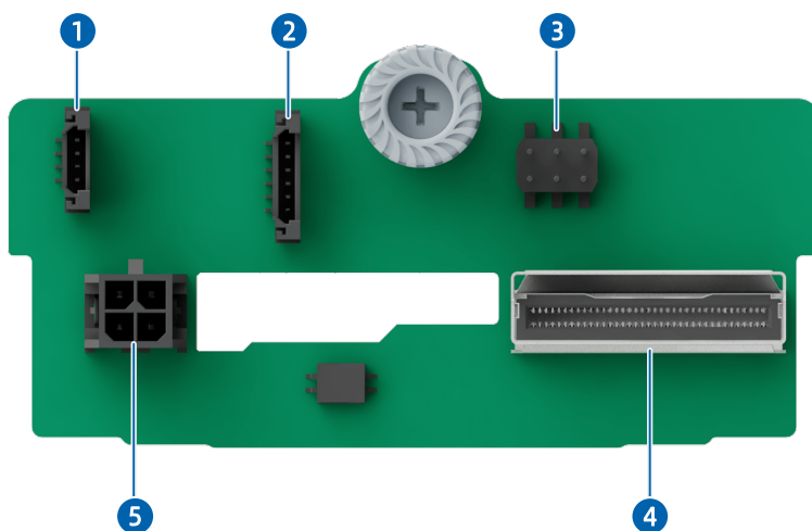
图 5-36 2 × 2.5 英寸 (NVMe) 硬盘背板
