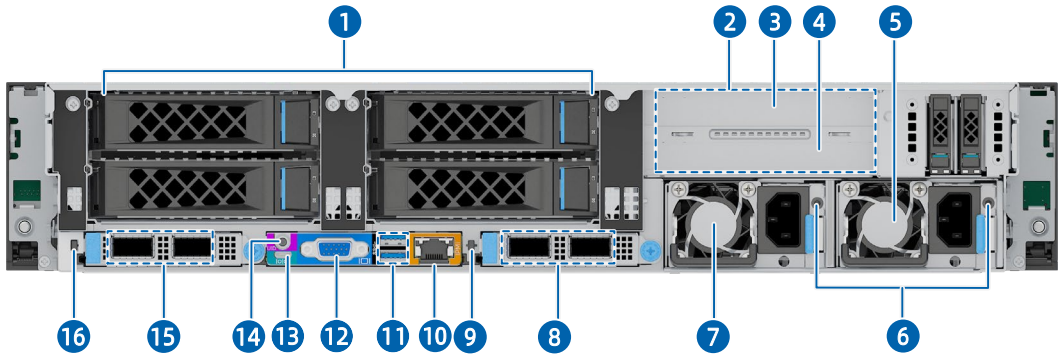
图 5-7 4 × 3.5 英寸硬盘+2 × PCIe 插槽配置后面板外观
