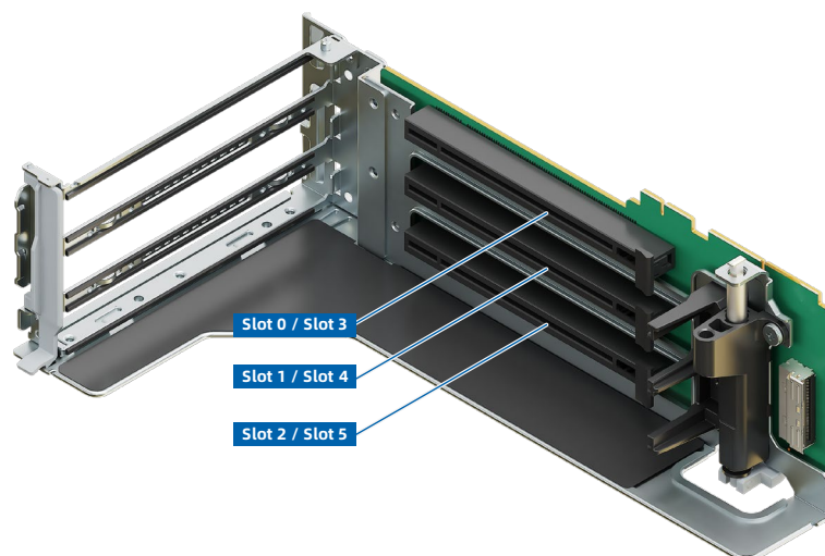
图 5-22 PCIe 转接卡模组 0/1 (3 个 x16 插槽)
