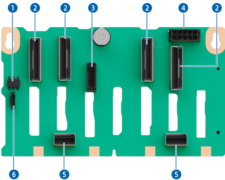
图 5-28 8 × 2.5 英寸（SAS/SATA/NVMe）硬盘背板
