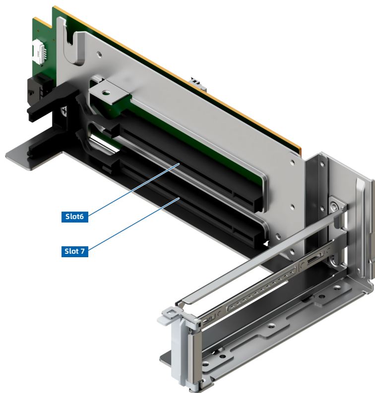
图 5-23 PCIe 转接卡模组 2 (2 个 x16 插槽)
