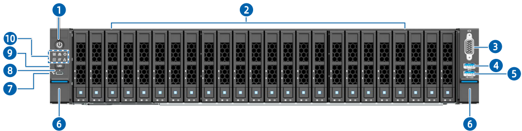
图 5-4 24 × E3.S SSD 配置前面板外观
