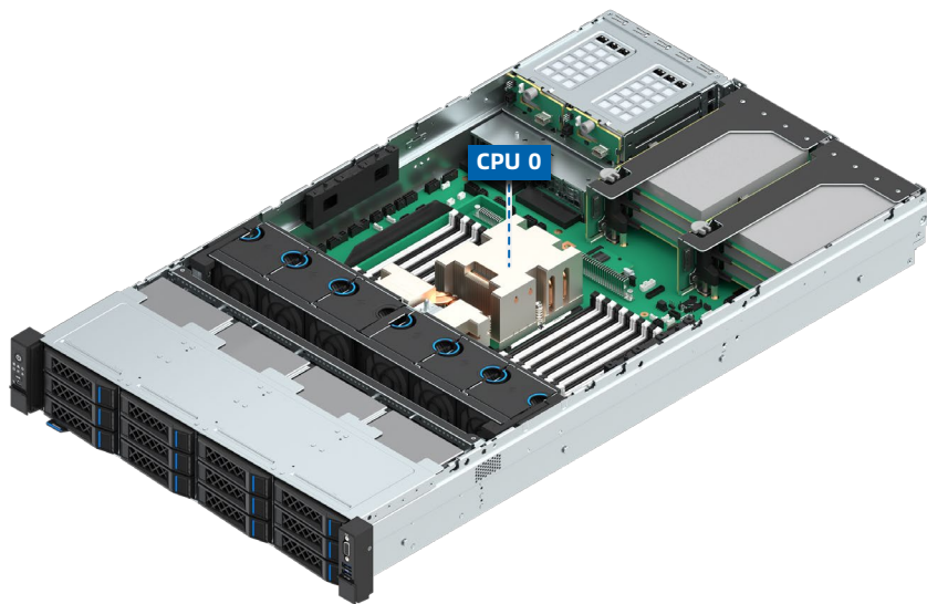
图 5-10 处理器位置
