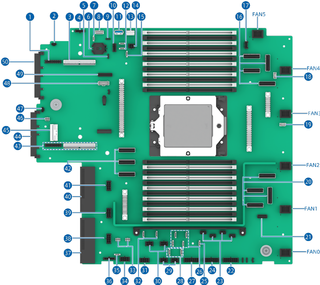
图 5-27 主板
