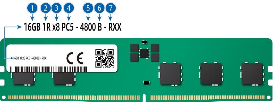
图 5-11 内存标识
