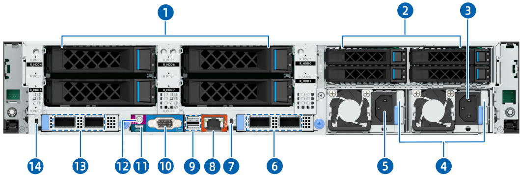
图 5-6 4 × 3.5 英寸硬盘+4 × 2.5 英寸硬盘配置后面板外观
