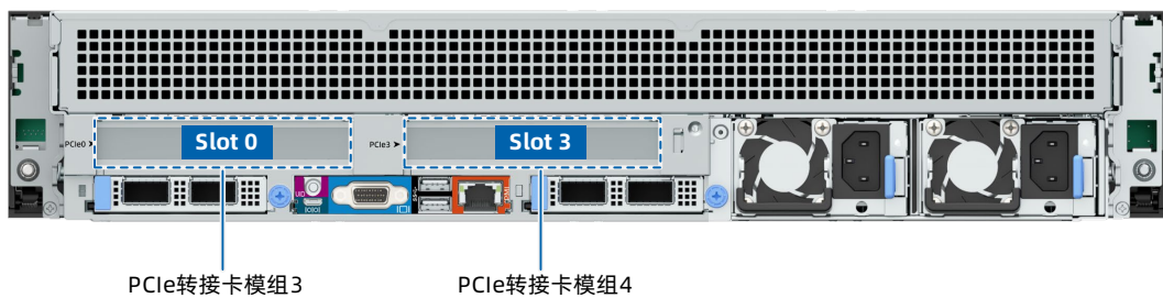
图 5-21 PCIe 插槽-2 × PCIe 插槽+4 × GPU 配置
