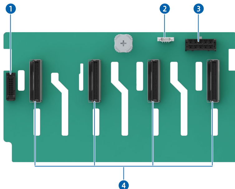
图 5-33 8 × E3.S SSD (E3.S SSD) 背板
