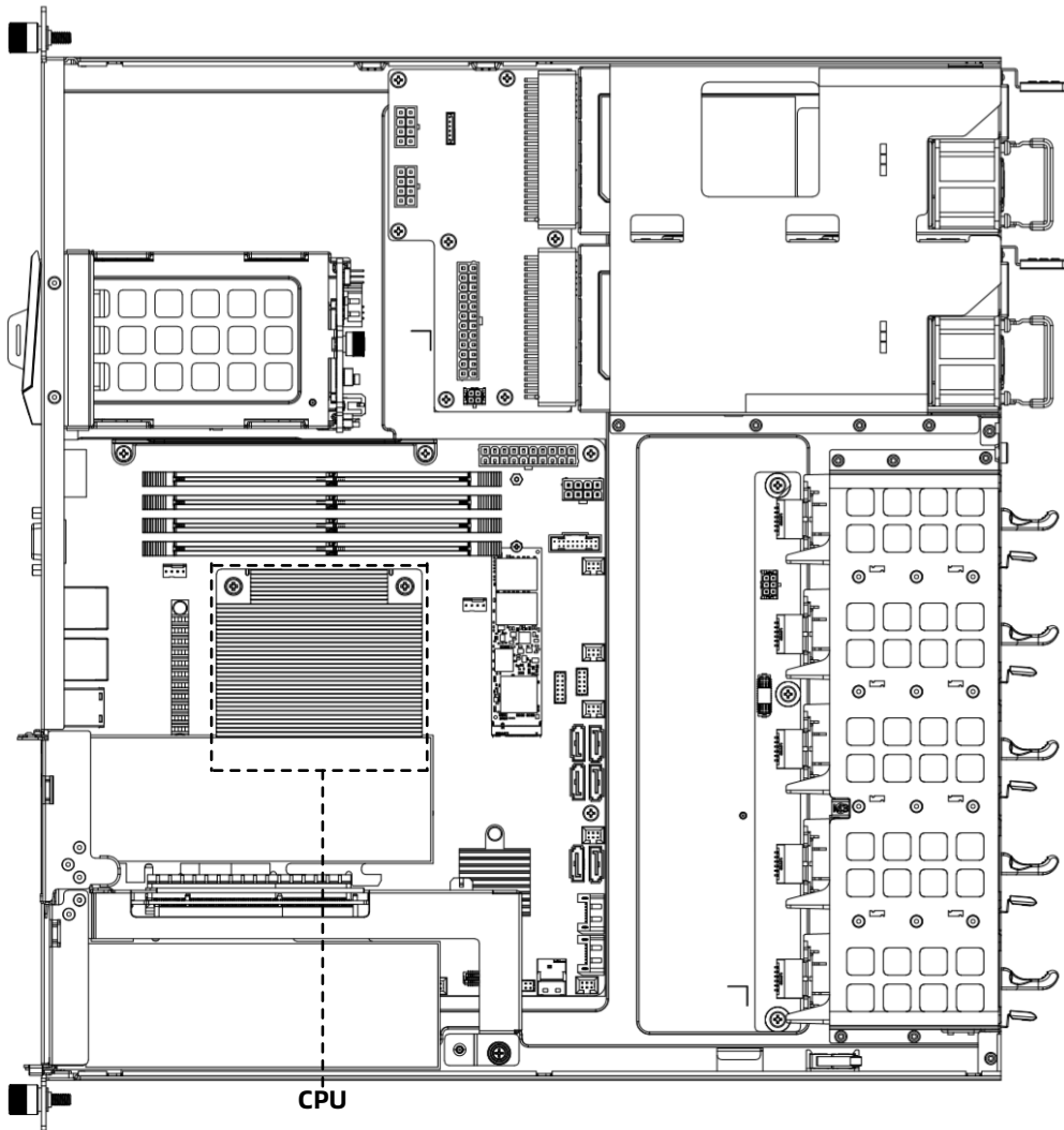
图 5-7 处理器位置
