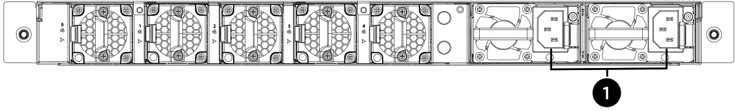
图 5-6 后面板接口
