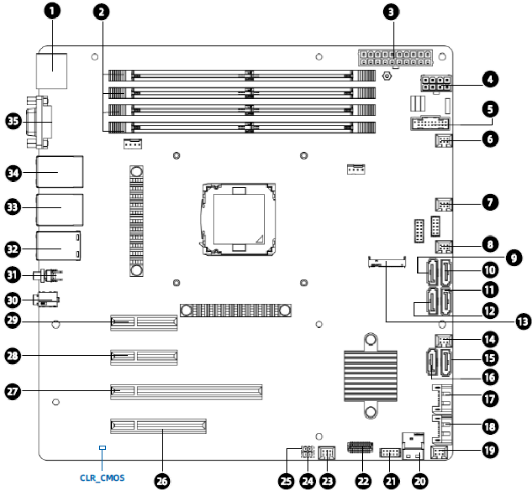
图 5-14 NE3120M5 主板
