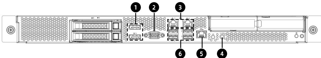
图 5-3 前面板接口
