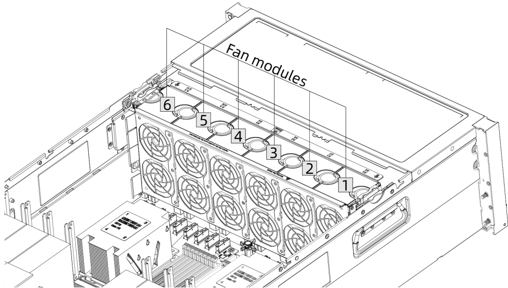
图 5-17 风扇模块的位置
