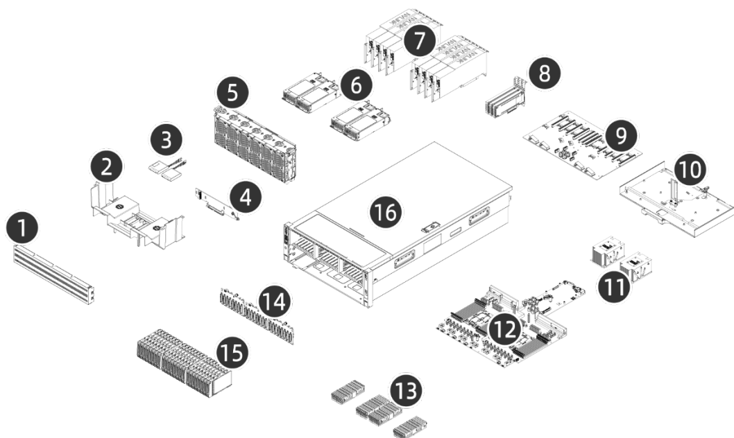
图 3-1 NF5468A5 物理结构 (示例: 24 × 2.5 英寸硬盘配置)
