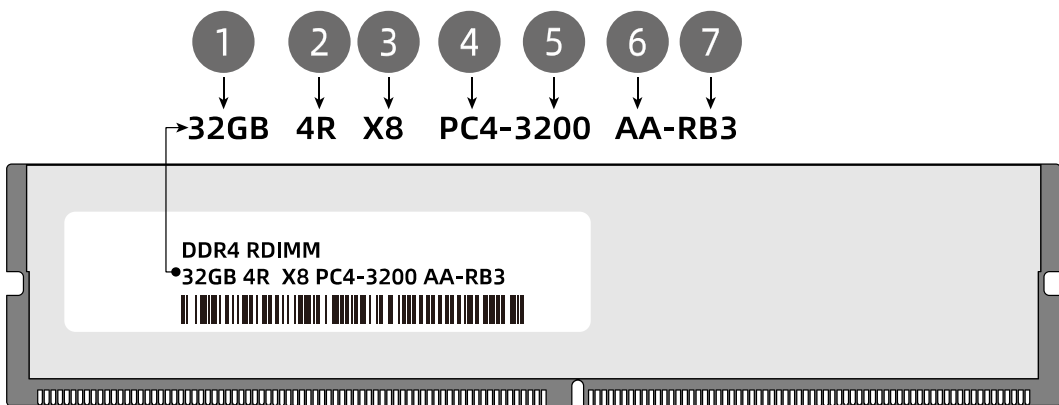
图 5-10 内存标识
