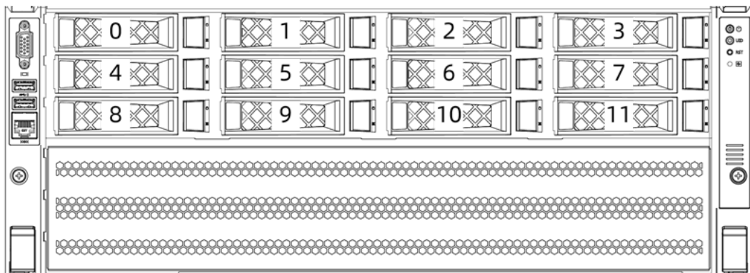
图 5-13 硬盘编号
