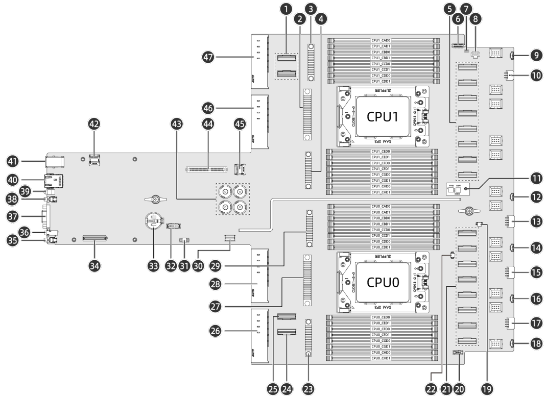
图 5-18 NF5468A5 主板
