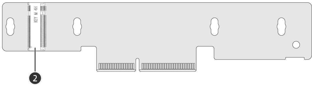
图 5-22 2 × M.2 直通配置 (2 × SATA/NVMe) 背板背面
