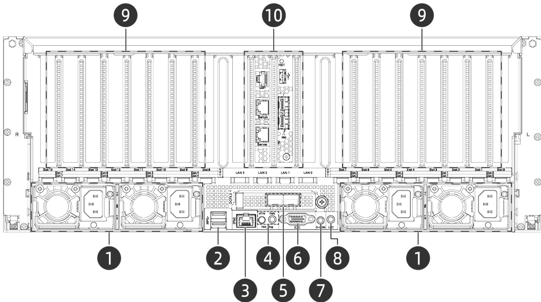
图 5-6 后面板外观
