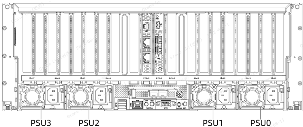
图 5-16 电源模块位置
