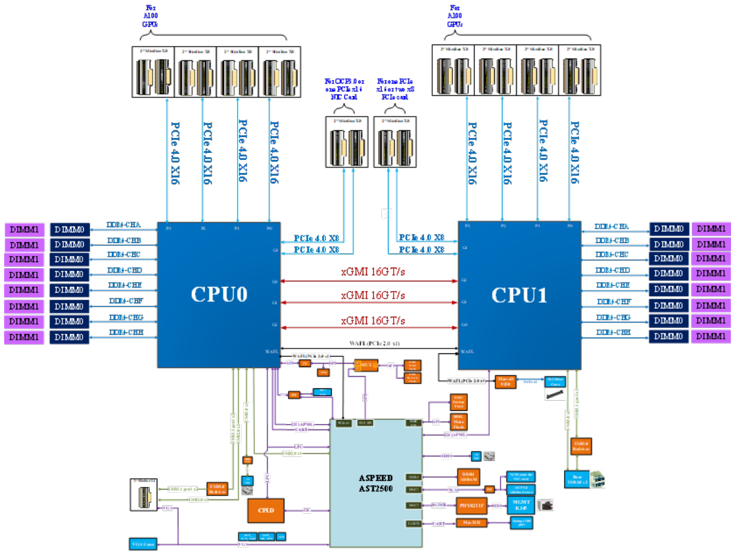
图 4-1 NF5468A5 逻辑结构
