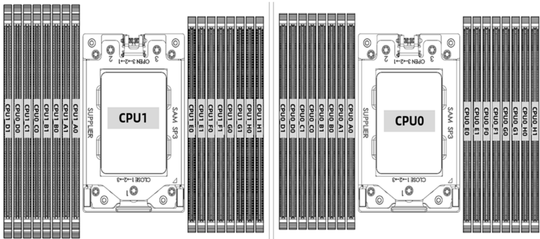
图 5-11 内存插槽位置
