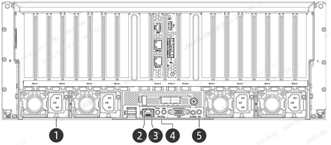
图 5-7 后面板指示灯
