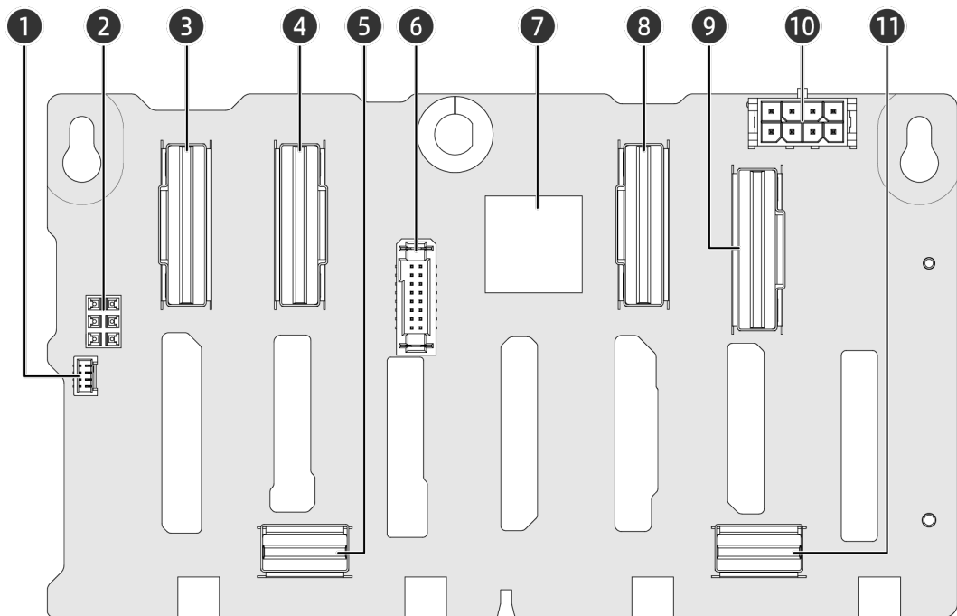
图 5-19 8 × 2.5 英寸硬盘直通配置 (8 × SAS/SATA/NVMe) 背板
