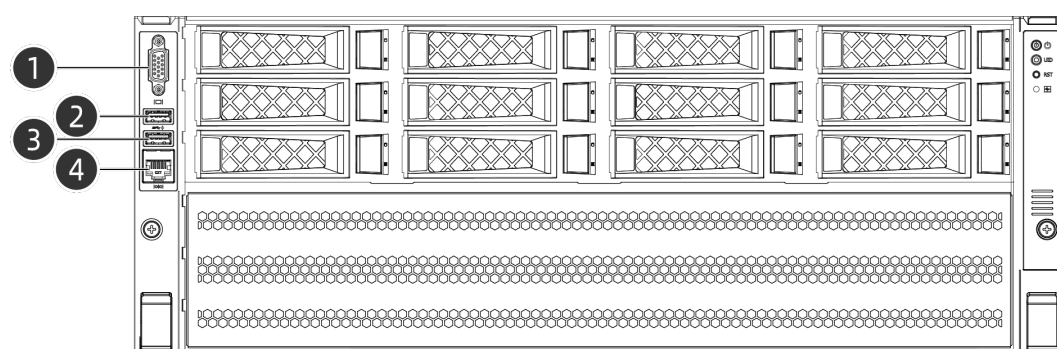
图 5-5 12 × 3.5 前面板接口
