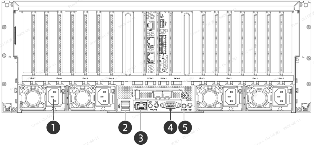
图 5-8 后面板接口
