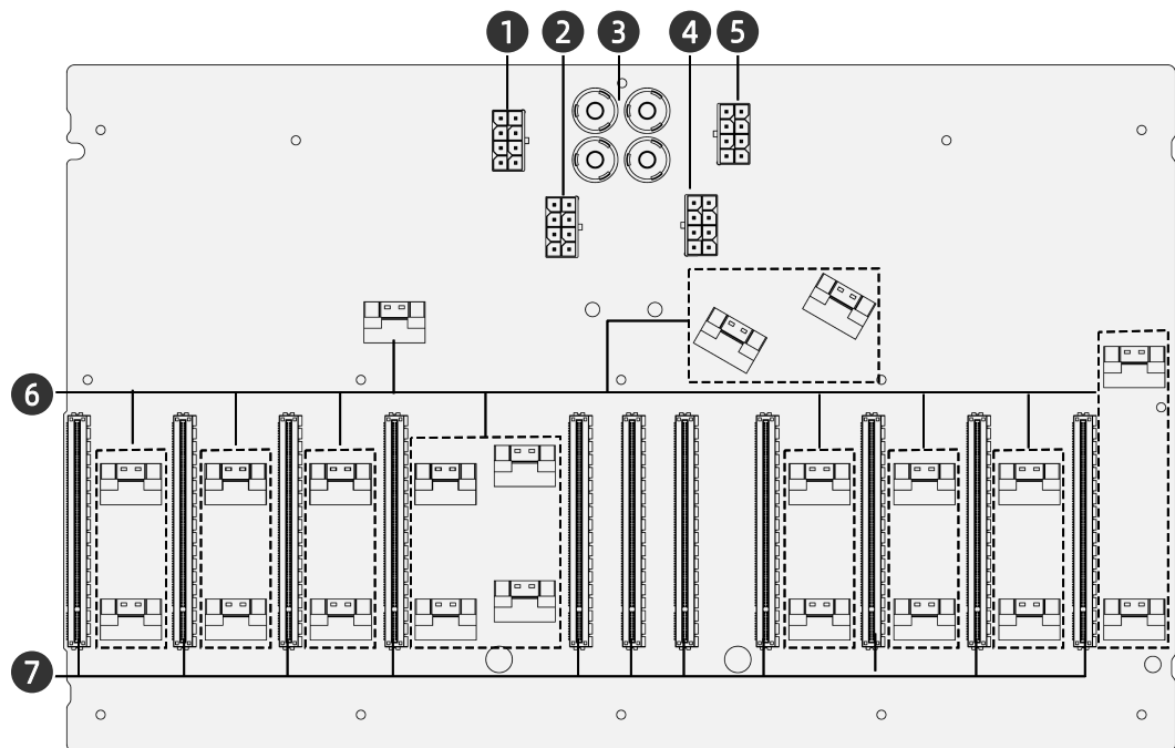
图 5-23 GPU 板布局图
