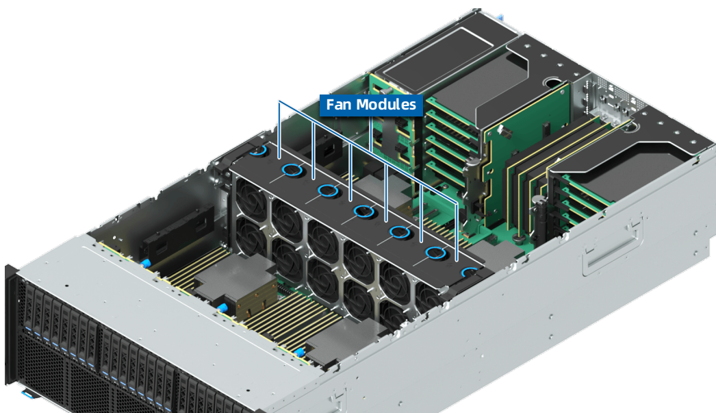
图 5-30 风扇模块的位置
