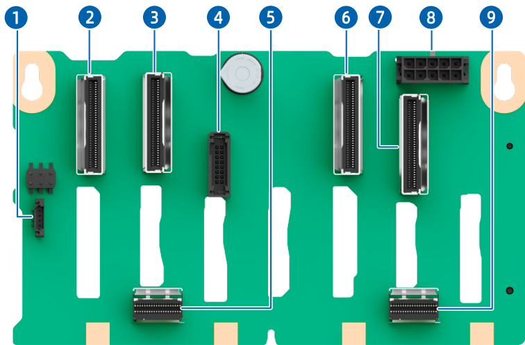
图 5-36 8 × 2.5 英寸硬盘背板
