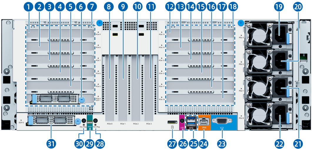
图 5-7 后面板外观
