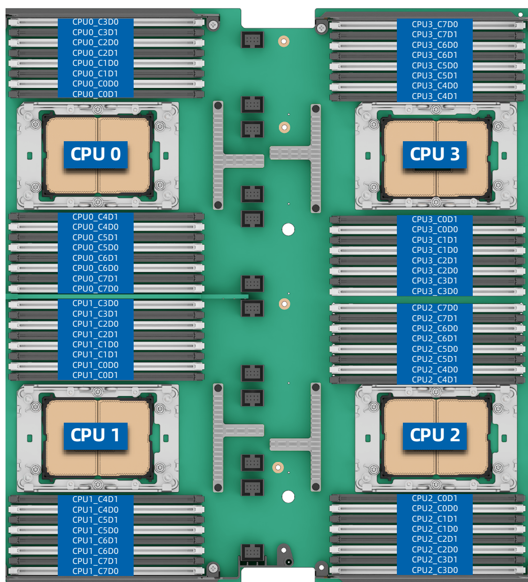
图 5-13 内存插槽位置
