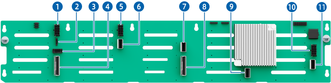
图 5-44 25 × 2.5 英寸硬盘背板
