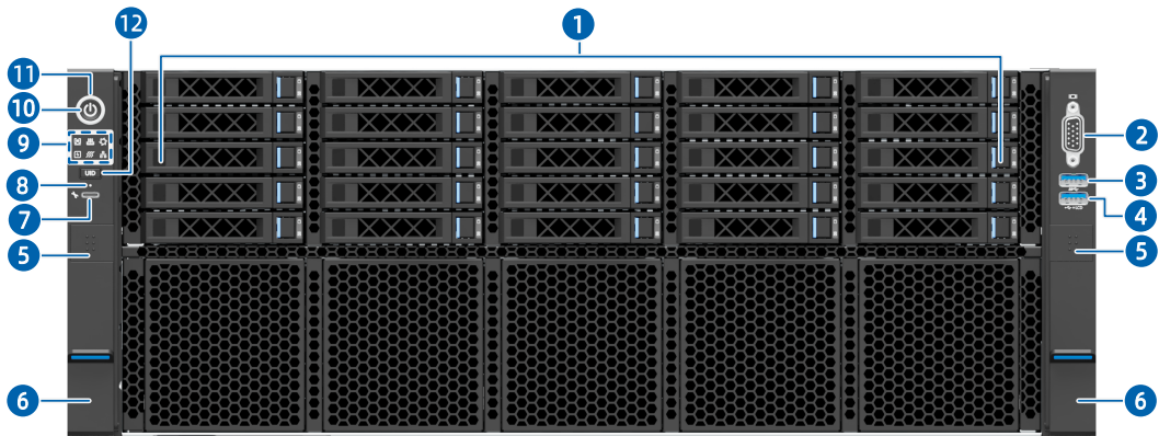
图 5-2 前面板外观
