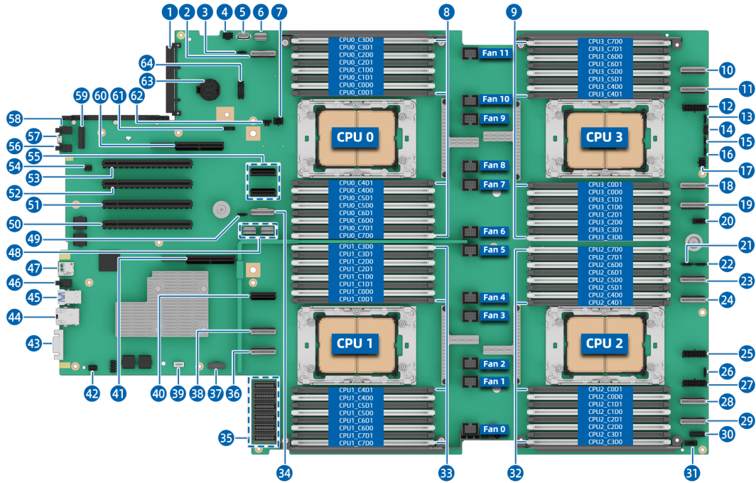
图 5-33 主板
