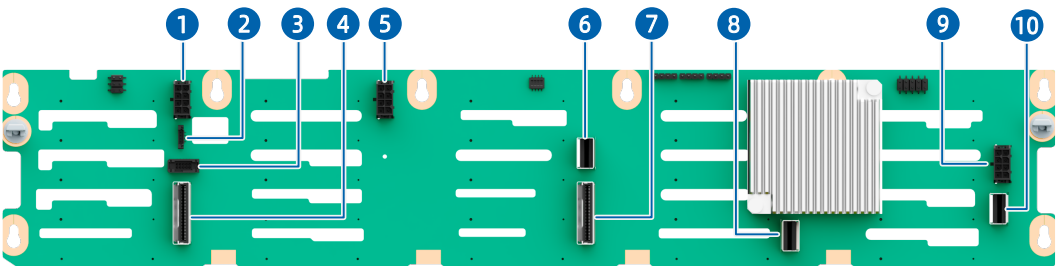
图 5-43 25 × 2.5 英寸硬盘背板
