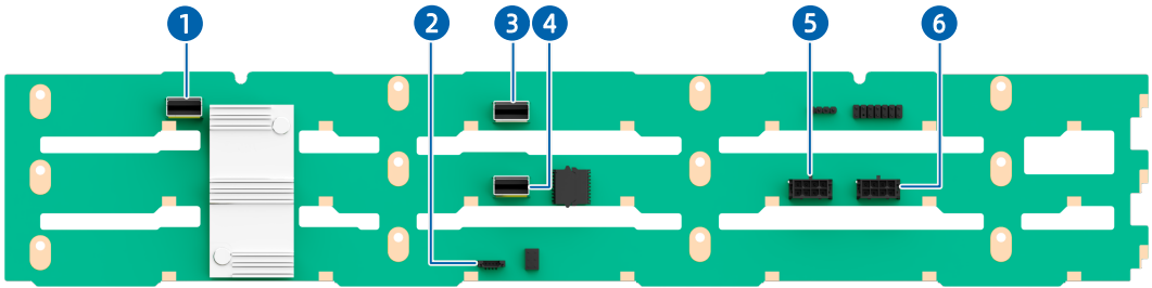
图 5-39 12 × 3.5 英寸硬盘背板
