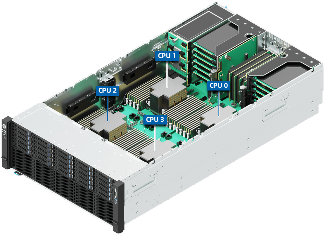
图 5-11 处理器位置
