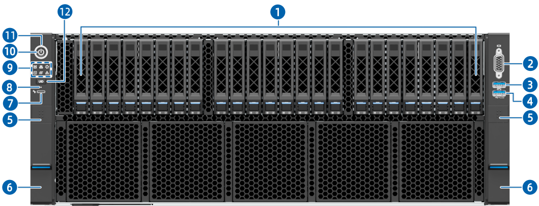
图 5-1 前面板外观
