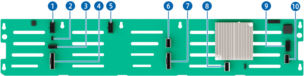
图 5-42 25 × 2.5 英寸硬盘背板
