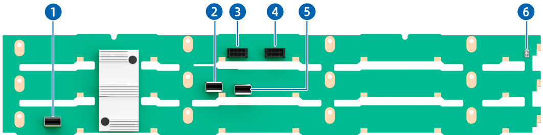
图 5-37 12 × 3.5 英寸硬盘背板
