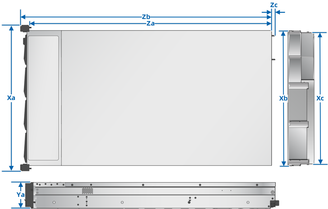
图 6-1 主机尺寸
