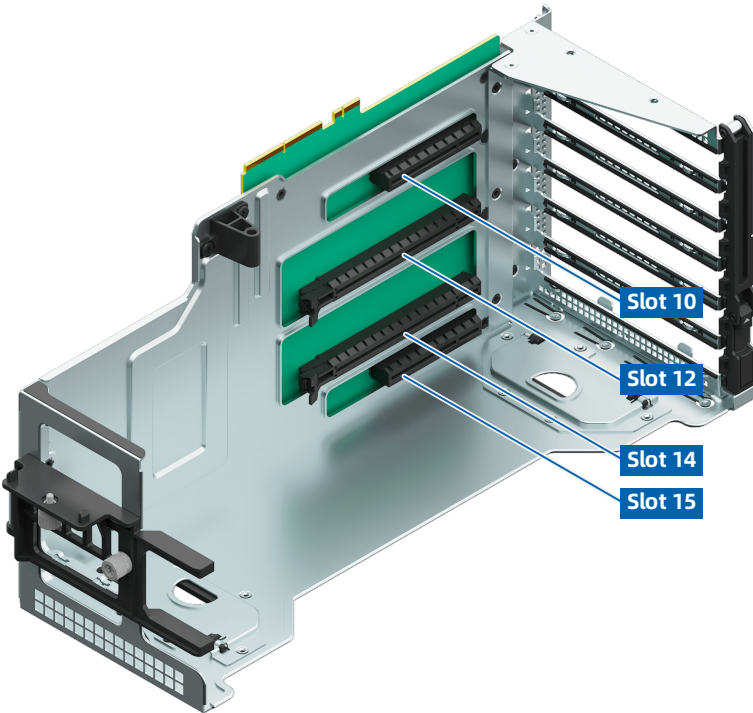
图 5-28 PCIe 转接卡模组 3-GPU（2 个 x16 插槽+2 个 x8 插槽）
