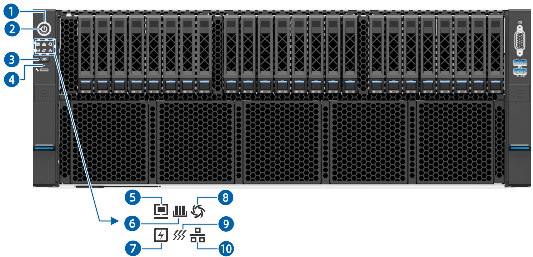
图 5-4 前面板按键与指示灯位置
