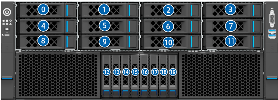
图 5-20 硬盘编号
