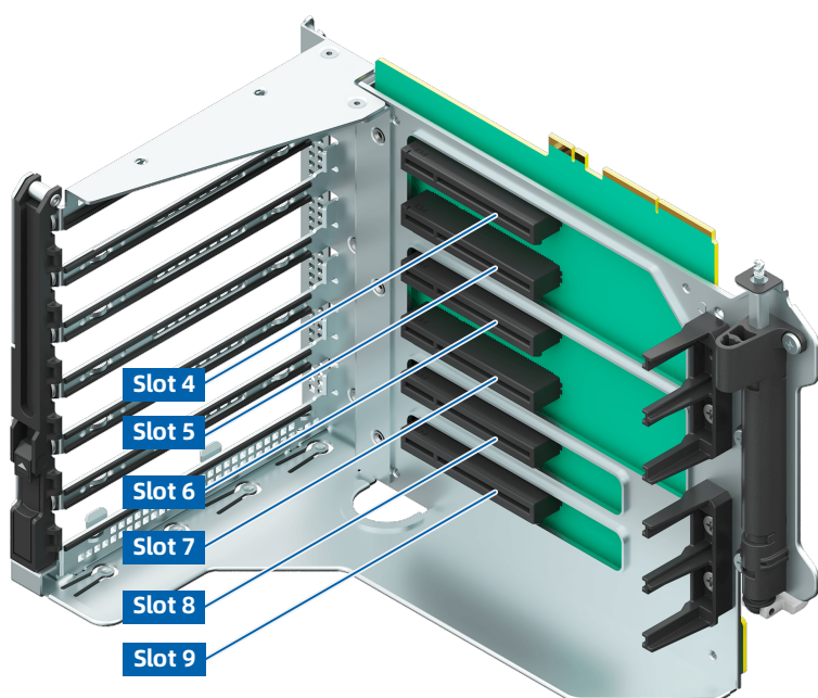
图 5-25 PCIe 转接卡模组 0（6 个 x8 插槽）
