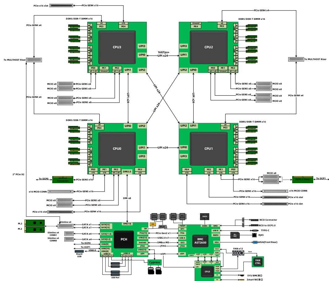
图 4-1 逻辑结构
