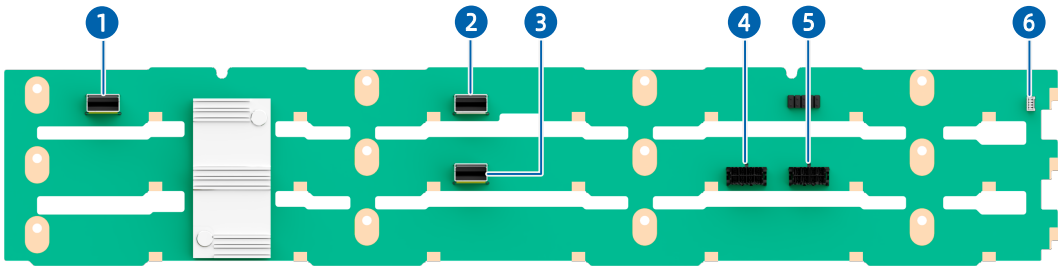
图 5-38 12 × 3.5 英寸硬盘背板
