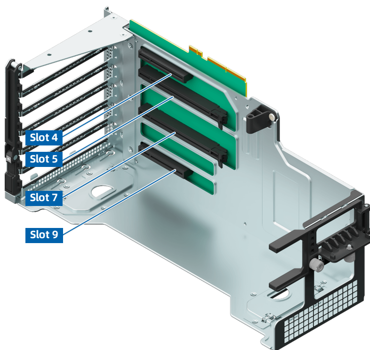
图 5-27 PCIe 转接卡模组 2-GPU (2 个 x16 插槽+2 个 x8 插槽)
