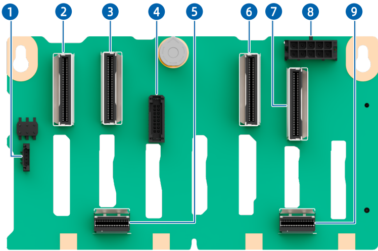
图 5-35 8 × 2.5 英寸硬盘背板
