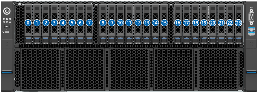
图 5-17 硬盘编号
