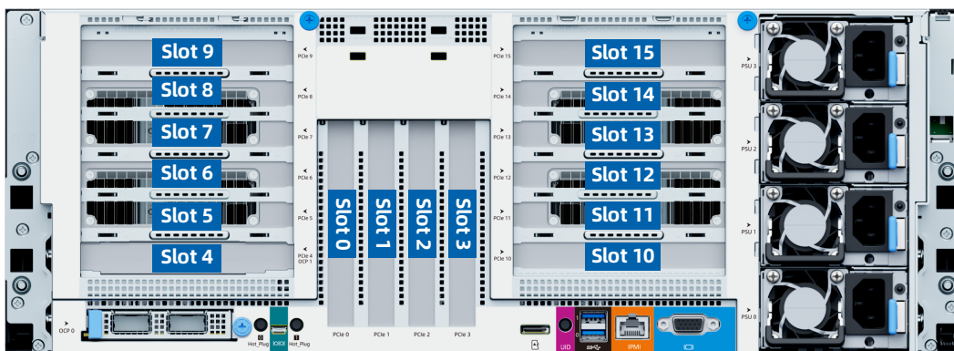
图 5-24 PCIe 插槽-GPU 配置
