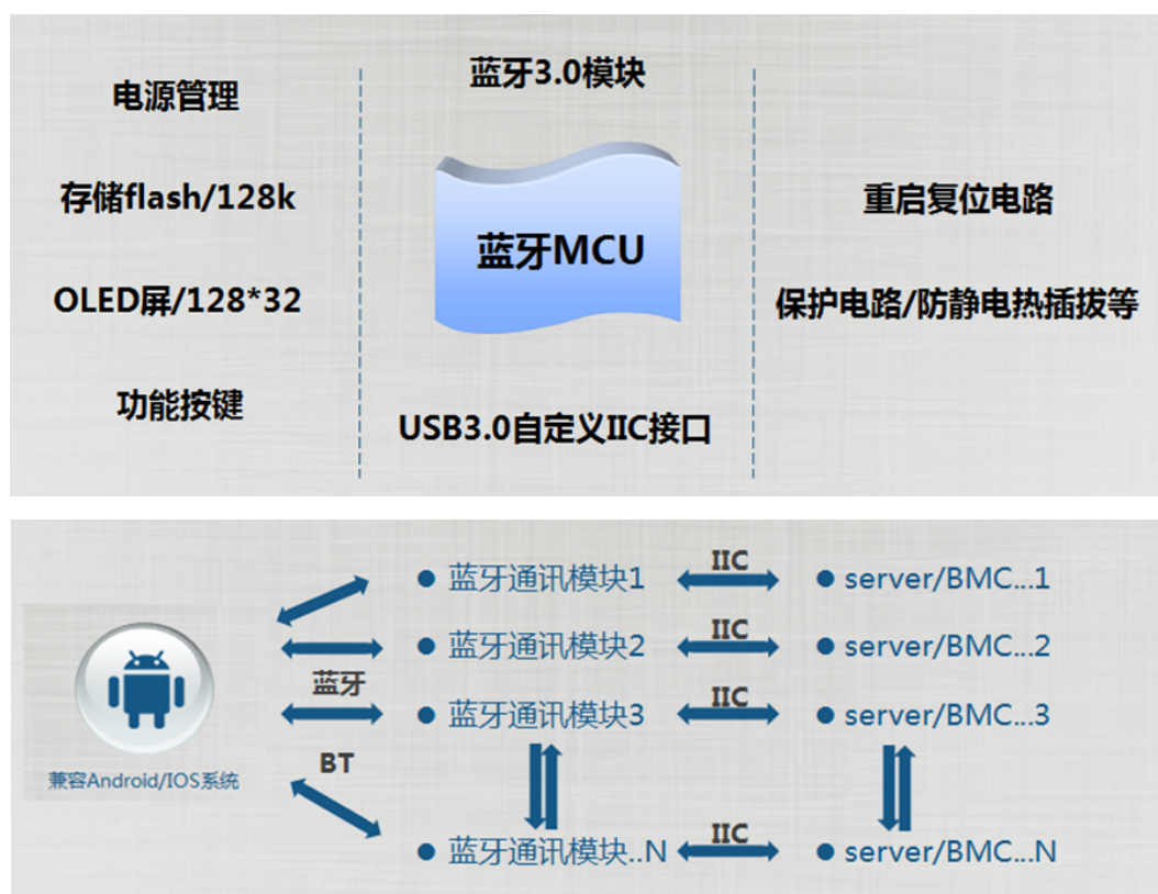
图 5-31 LCD 子系统工作原理
