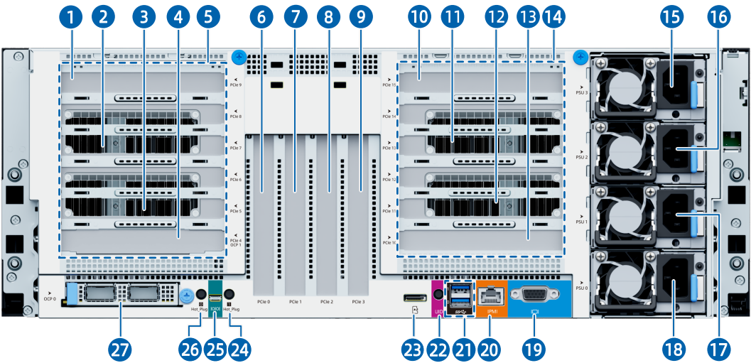
图 5-8 后面板外观
