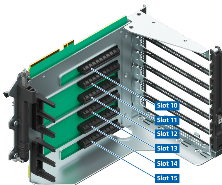
图 5-26 PCIe 转接卡模组 1 (6 个 x8 插槽)
