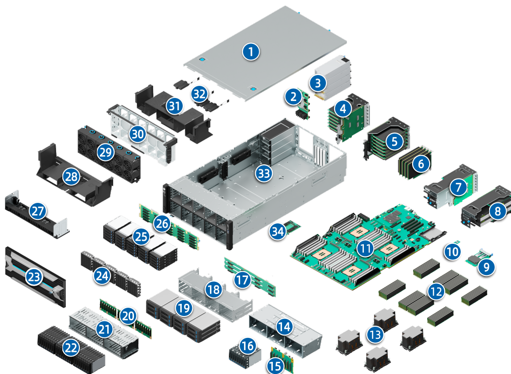
图 3-1 产品爆炸图
