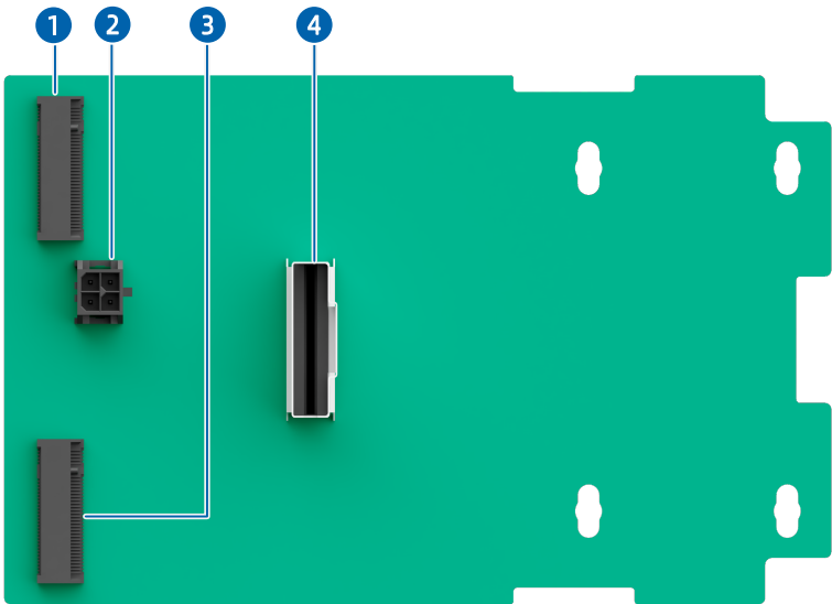
图 5-45 2 × M.2 硬盘背板
