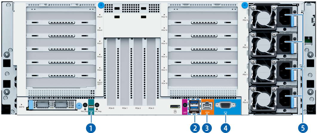
图 5-10 后面板接口位置
