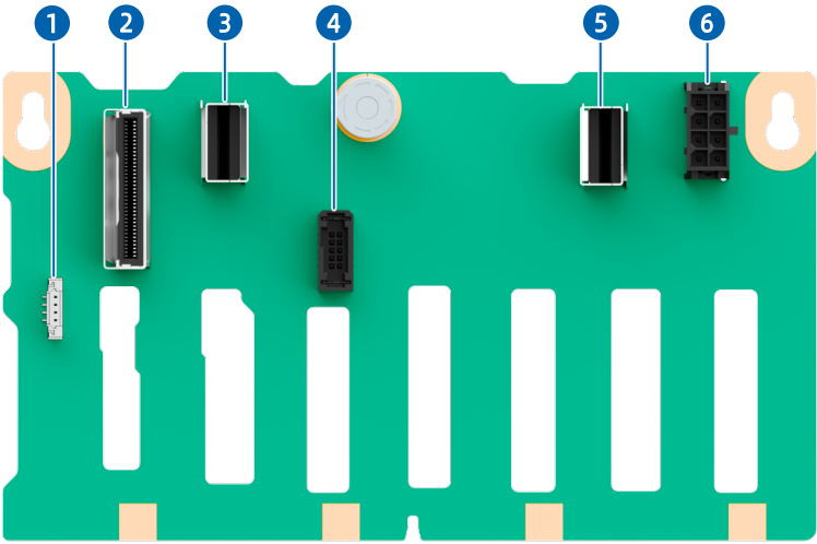
图 5-34 8 × 2.5 英寸硬盘背板
