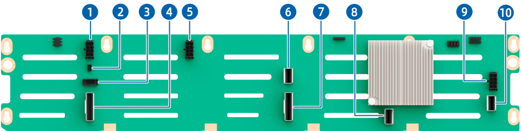
图 5-41 25 × 2.5 英寸硬盘背板
