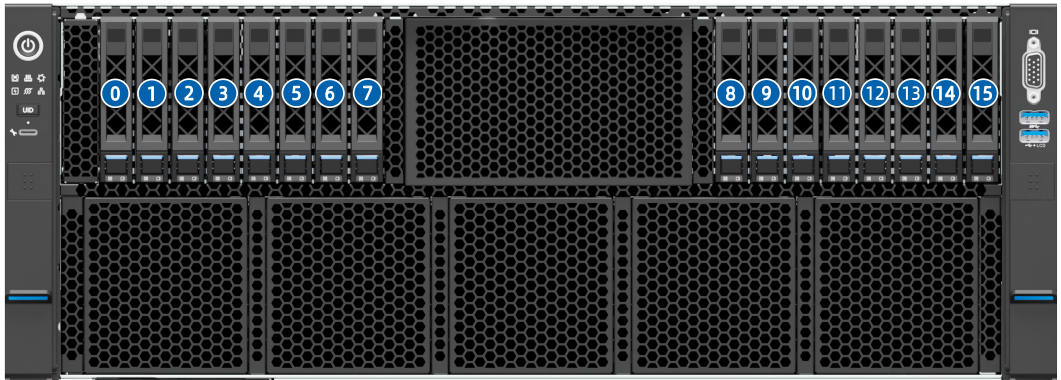
图 5-16 硬盘编号
