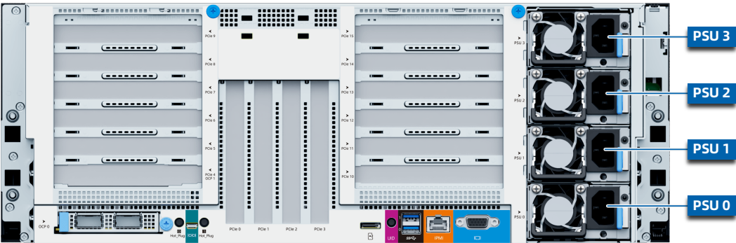
图 5-29 电源模块位置
