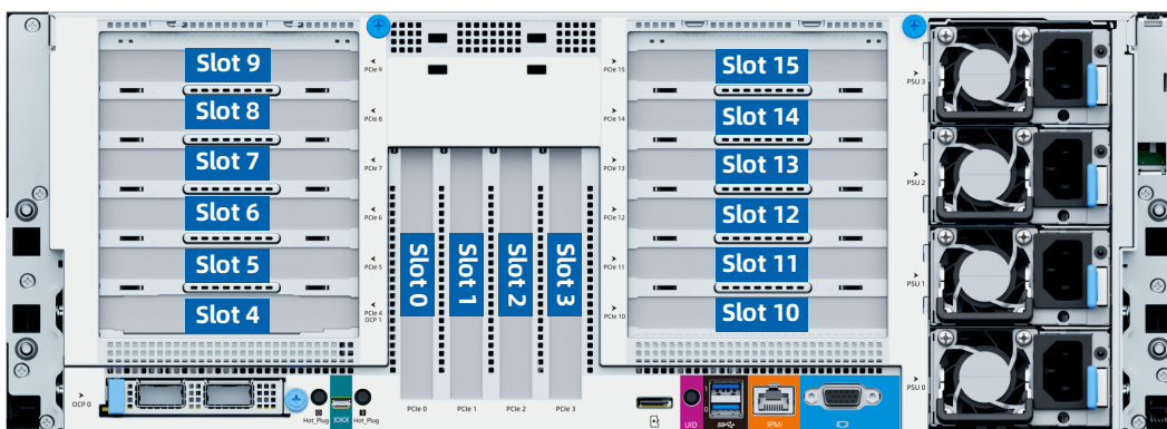
图 5-23 PCIe 插槽-普通配置
