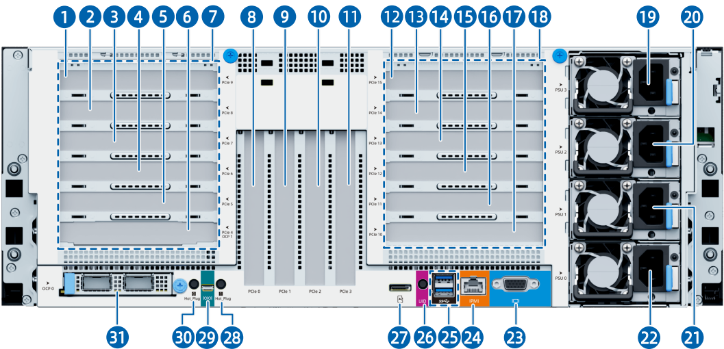
图 5-6 后面板外观
