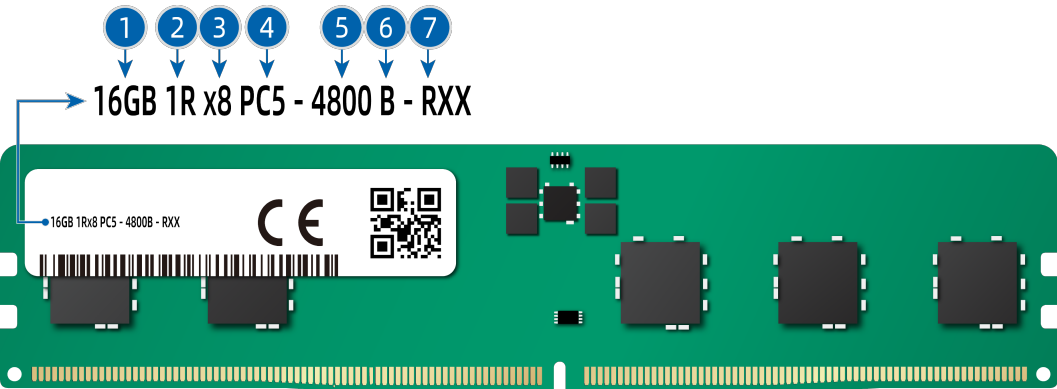
图 5-12 内存标识
