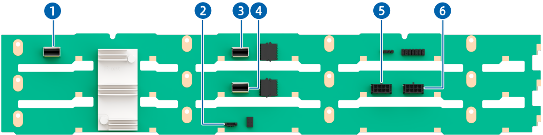
图 5-40 12 × 3.5 英寸硬盘背板
