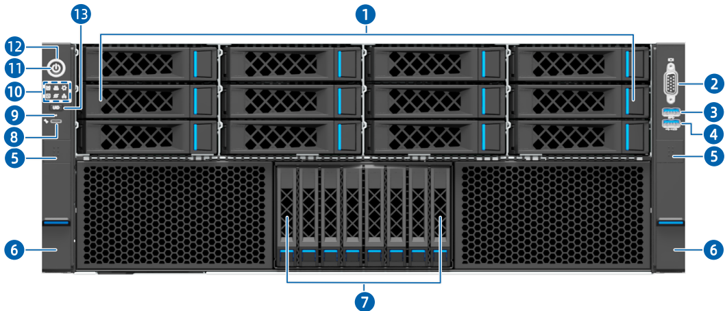
图 5-3 前面板外观
